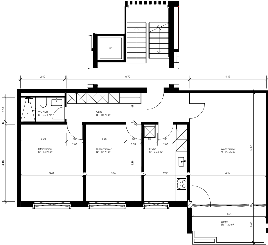
MST 1:100
