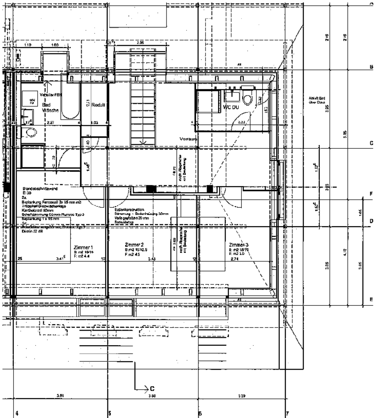
Dachgeschoss m 1:50
