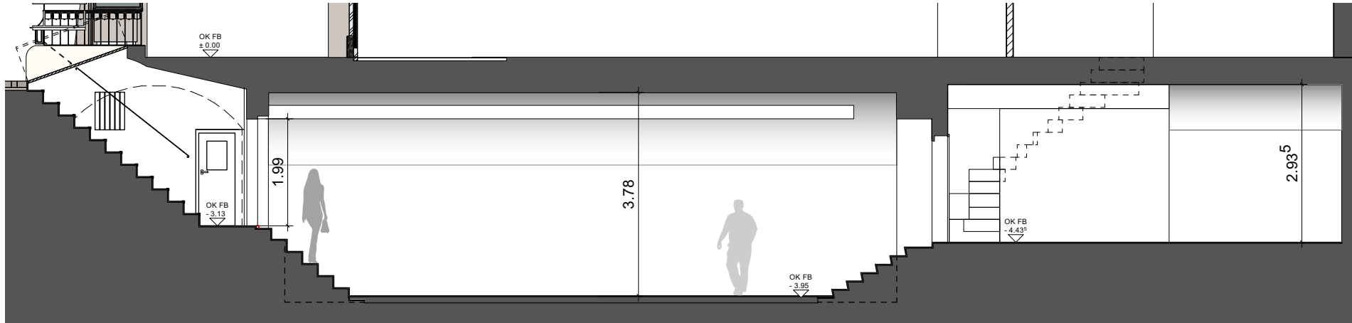
Schnitt A-A
