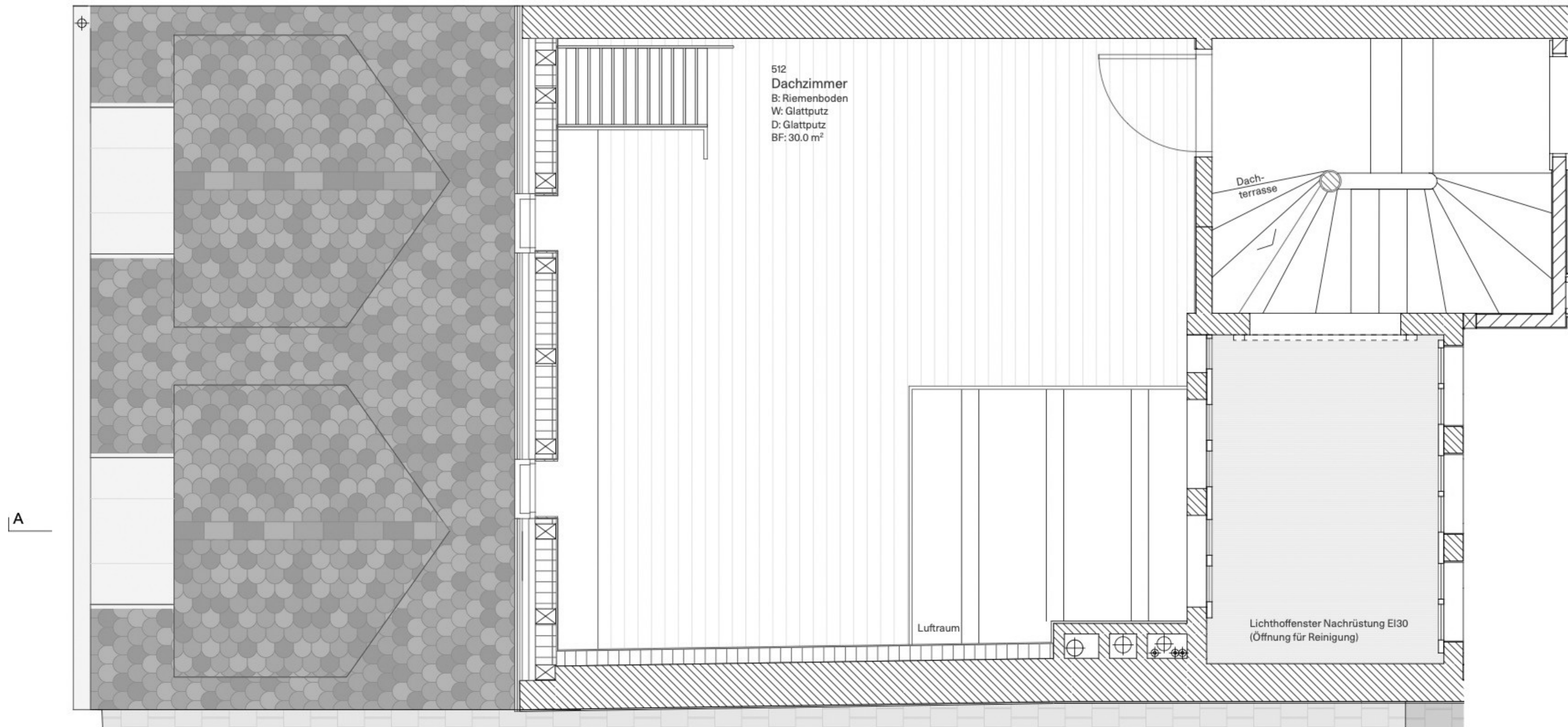
GRUNDRISS
