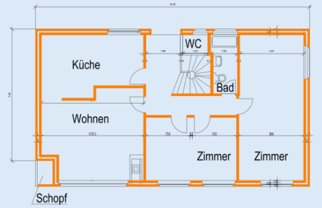
Grundriss Erdgeschoss
