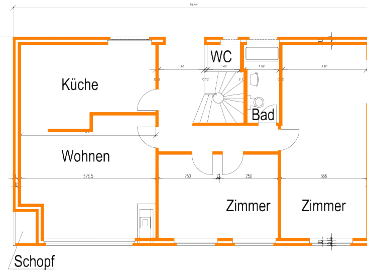
Grundriss Erdgeschoss
