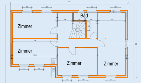
Grundriss Dachgeschoss
