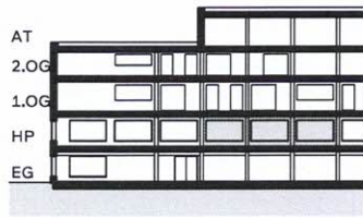
Schnitt
