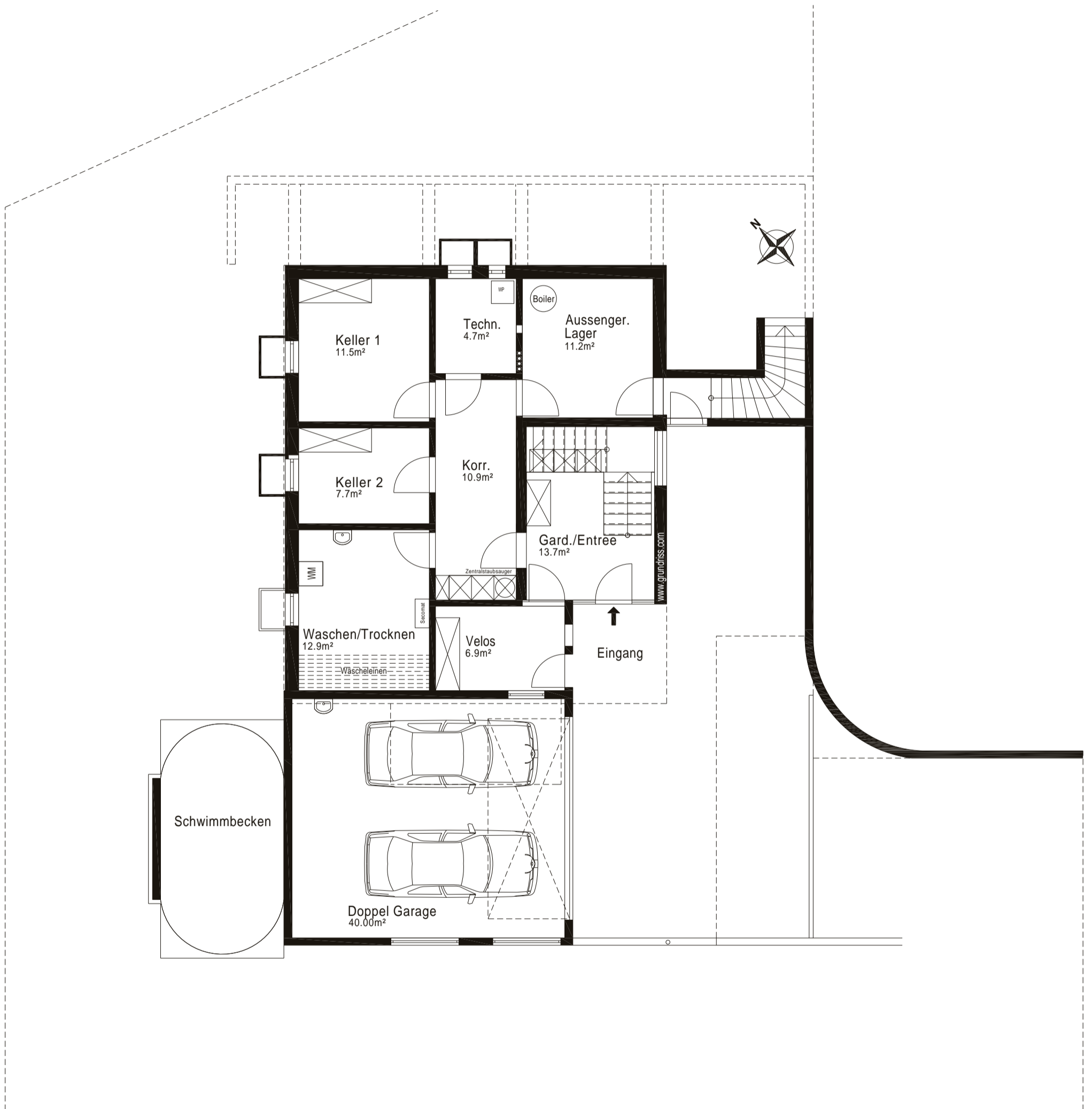
Untergeschoss
