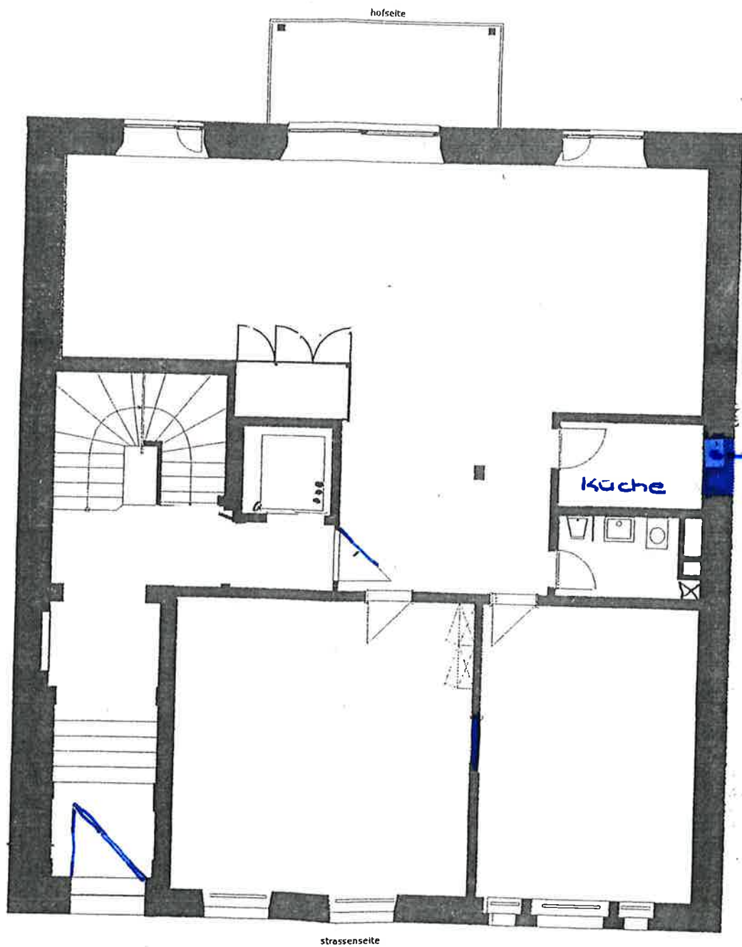
ERDGESCHOSS 1: 100
