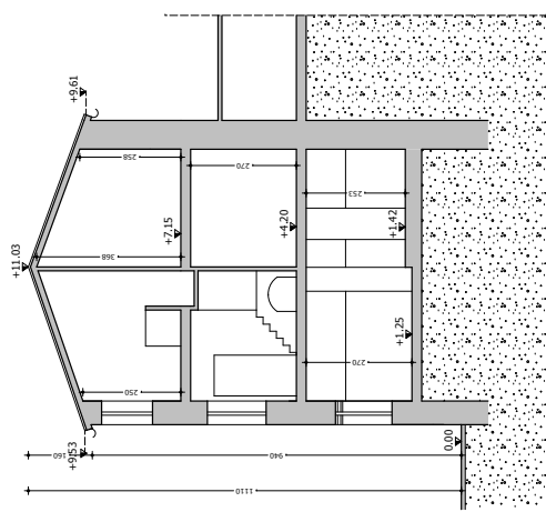
SEZIONE B-B SCALA 1:100
