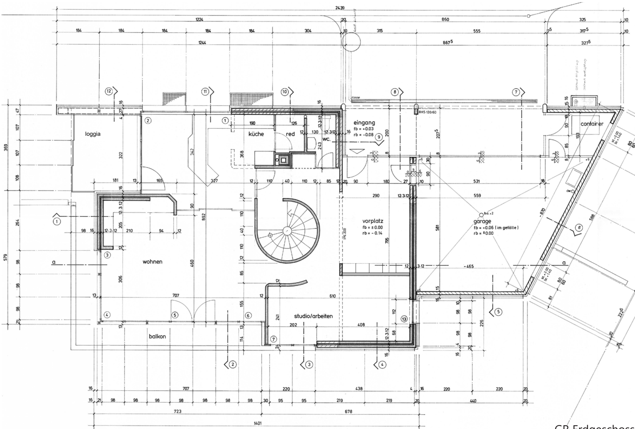
GR Erdgeschoss
