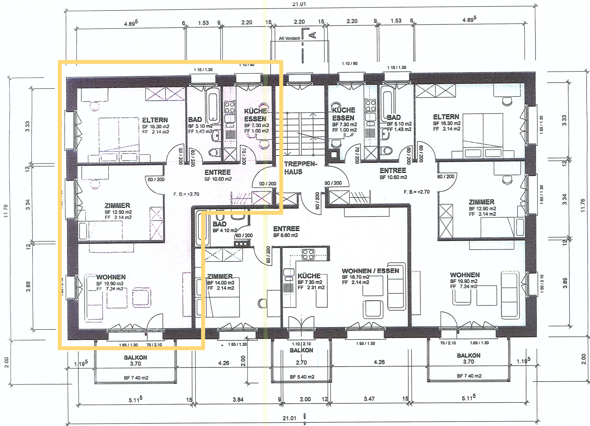
GRUNDRISS 1.OBERGESCHOSS
