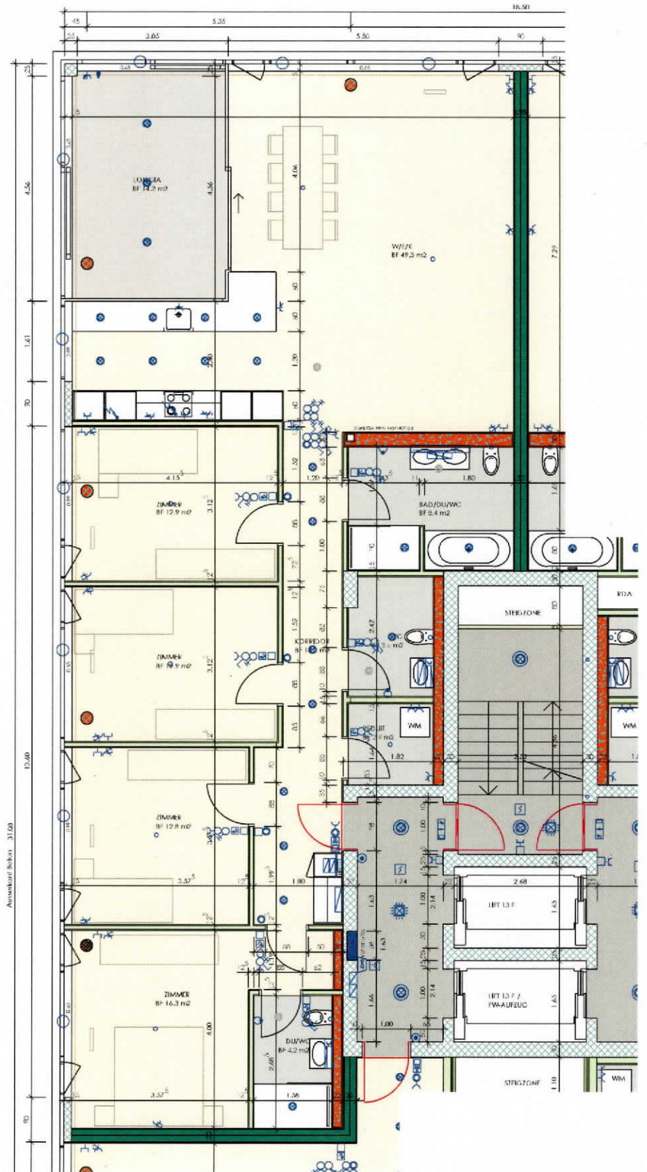
GRUNDRISS
