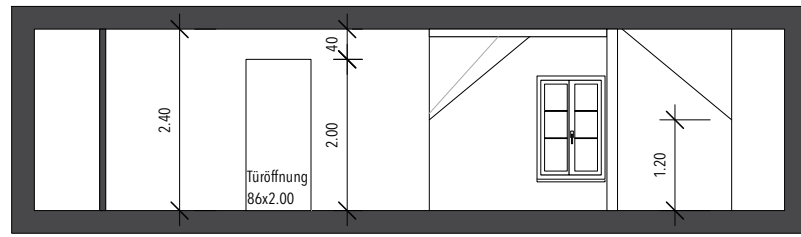
Schnitt A-A Dachgeschoss
