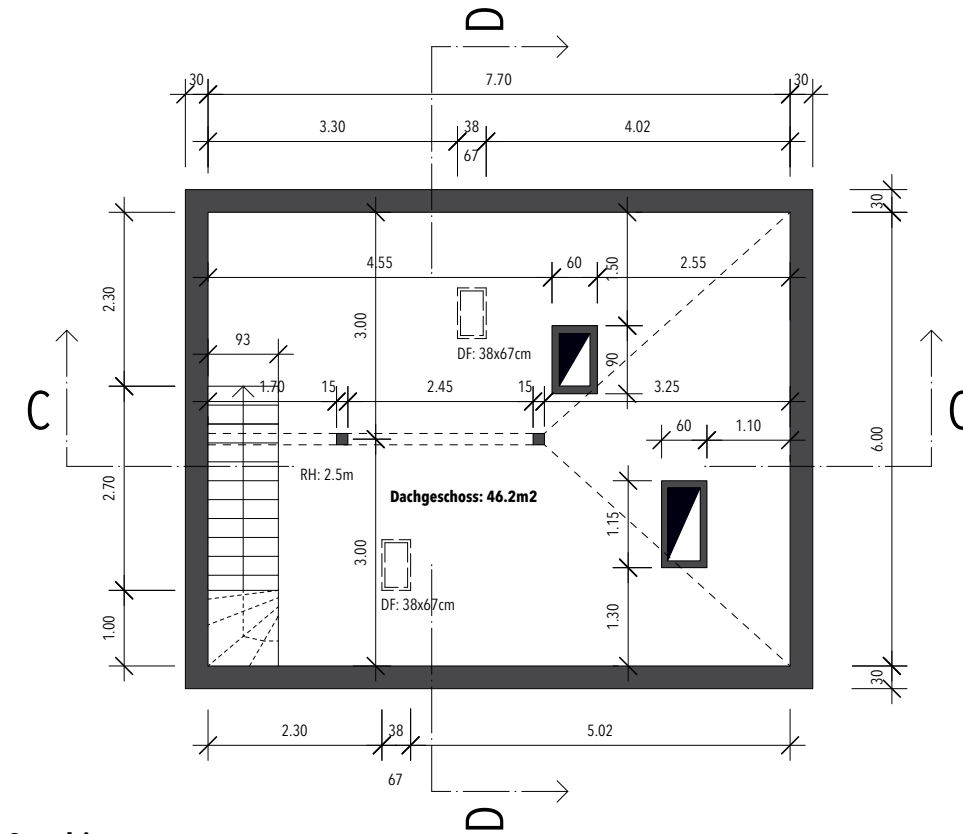
Grundriss Dachgeschoss
