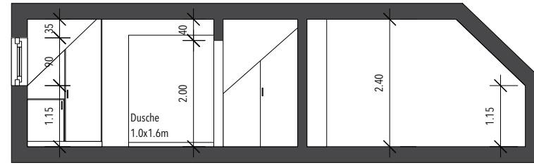
Schnitt B-B Dachgeschoss
