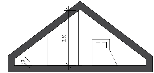
Schnitt D-D Dachgeschoss
