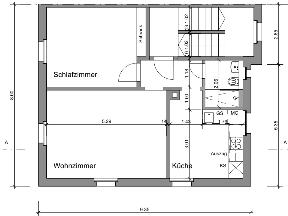
1.OG 1:100
