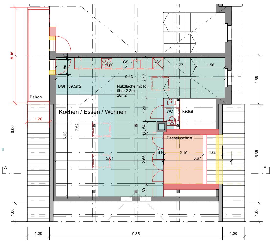
DG 1:100
