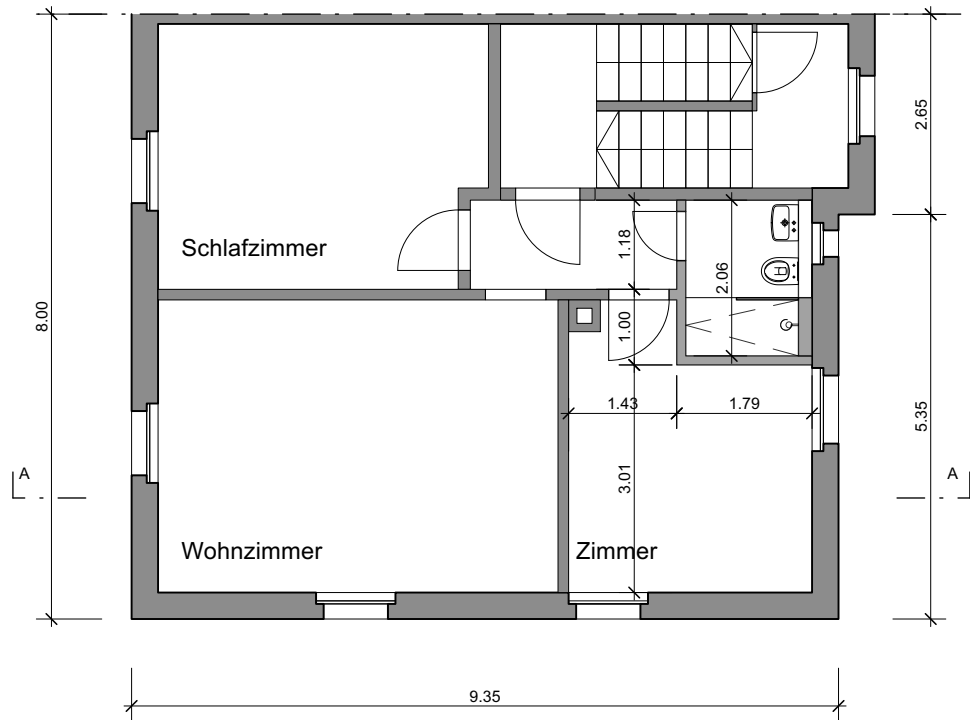
2.OG 1:100
