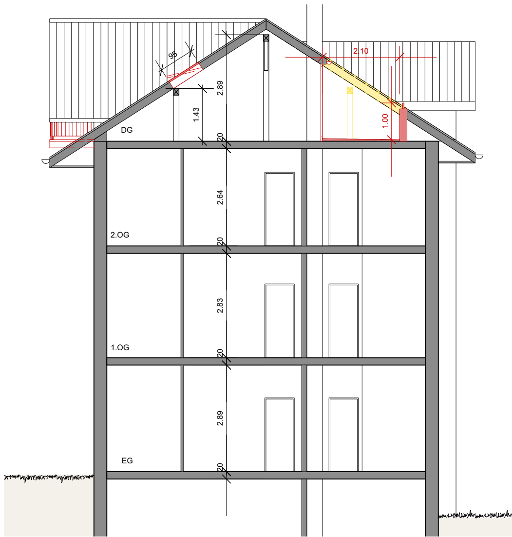
Schnitt A - A 1:100
