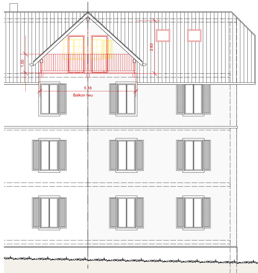
Südfassade 1:100
