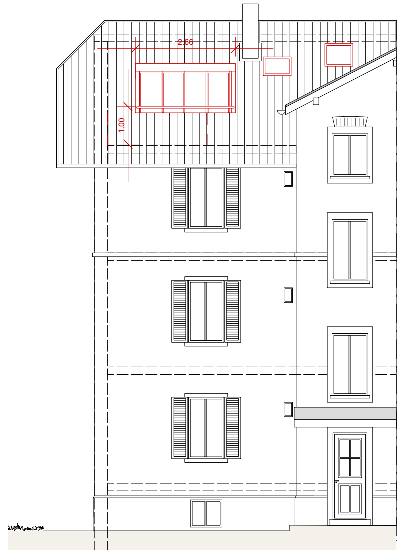
Nordfassade 1:100
