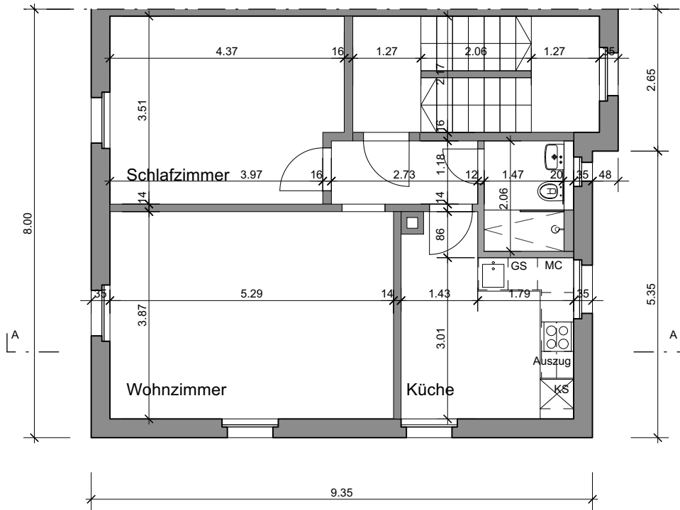
EG 1:100
