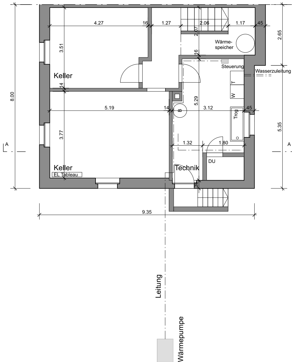
Keller 1:100
