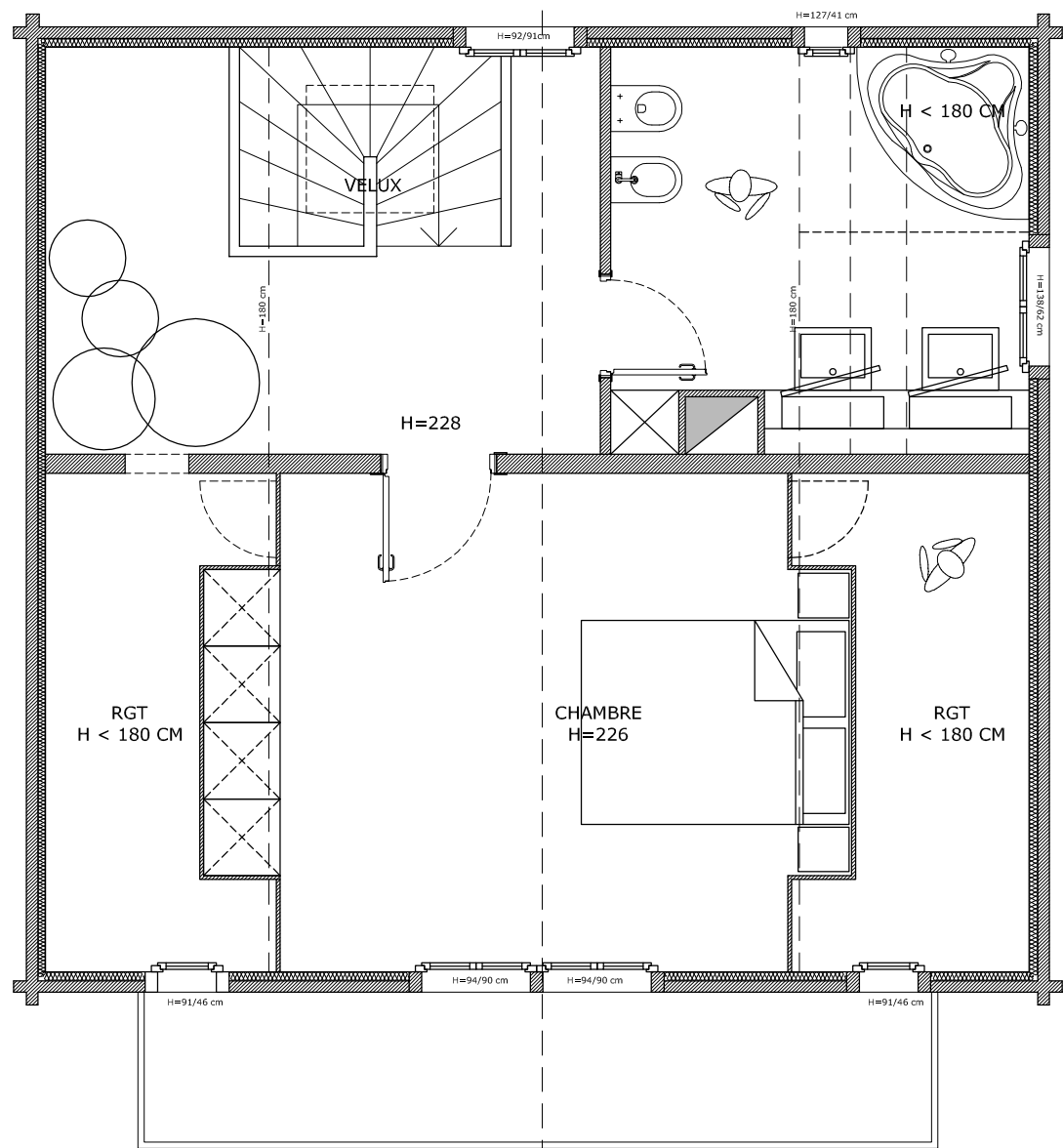
PLAN 2eme - hors ech.
