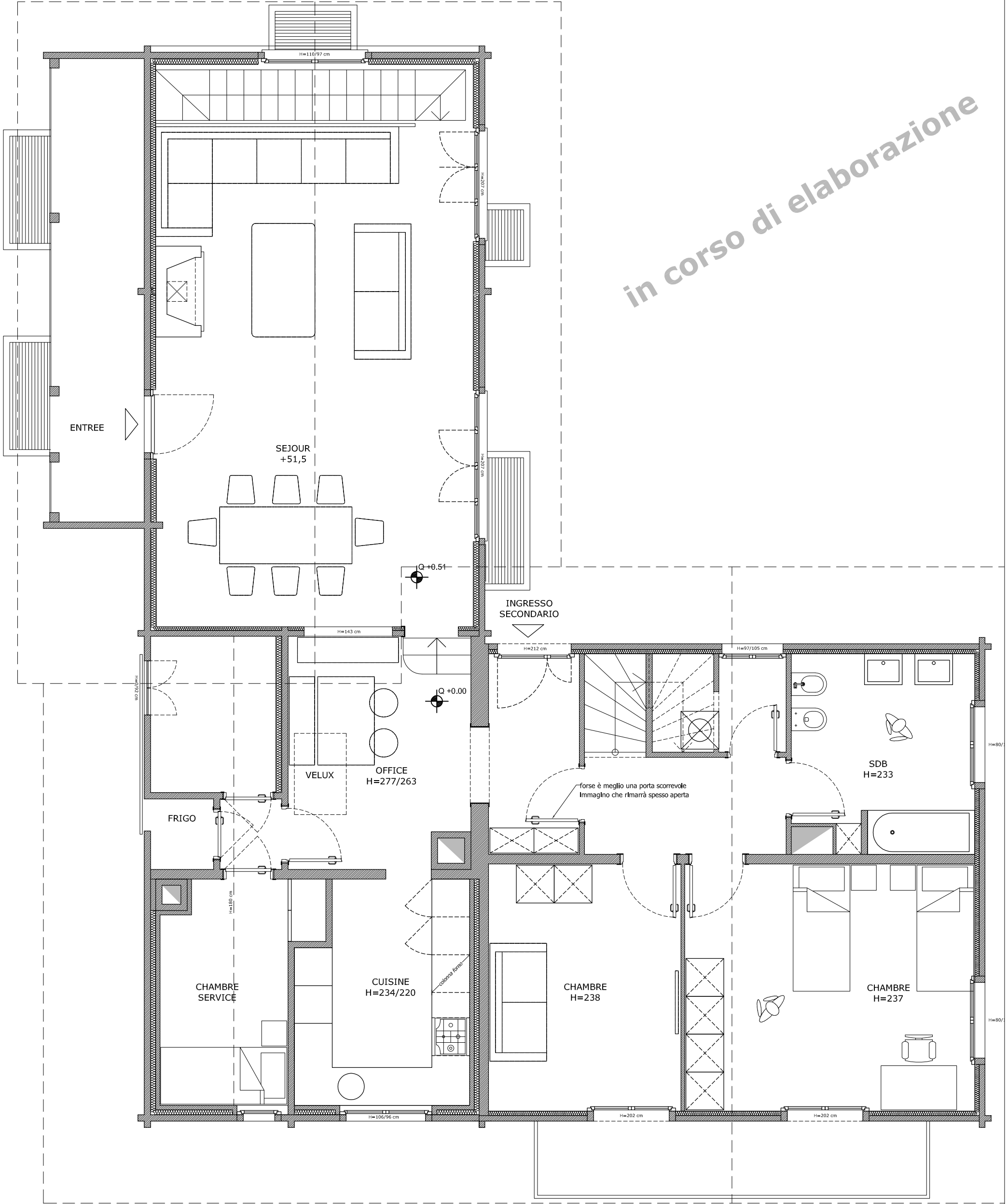
PLAN 1er - hors ech.
