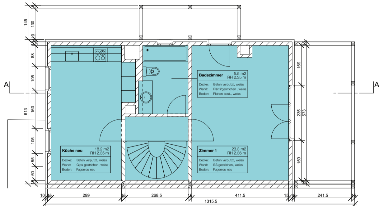
OBERGESCHOSS
