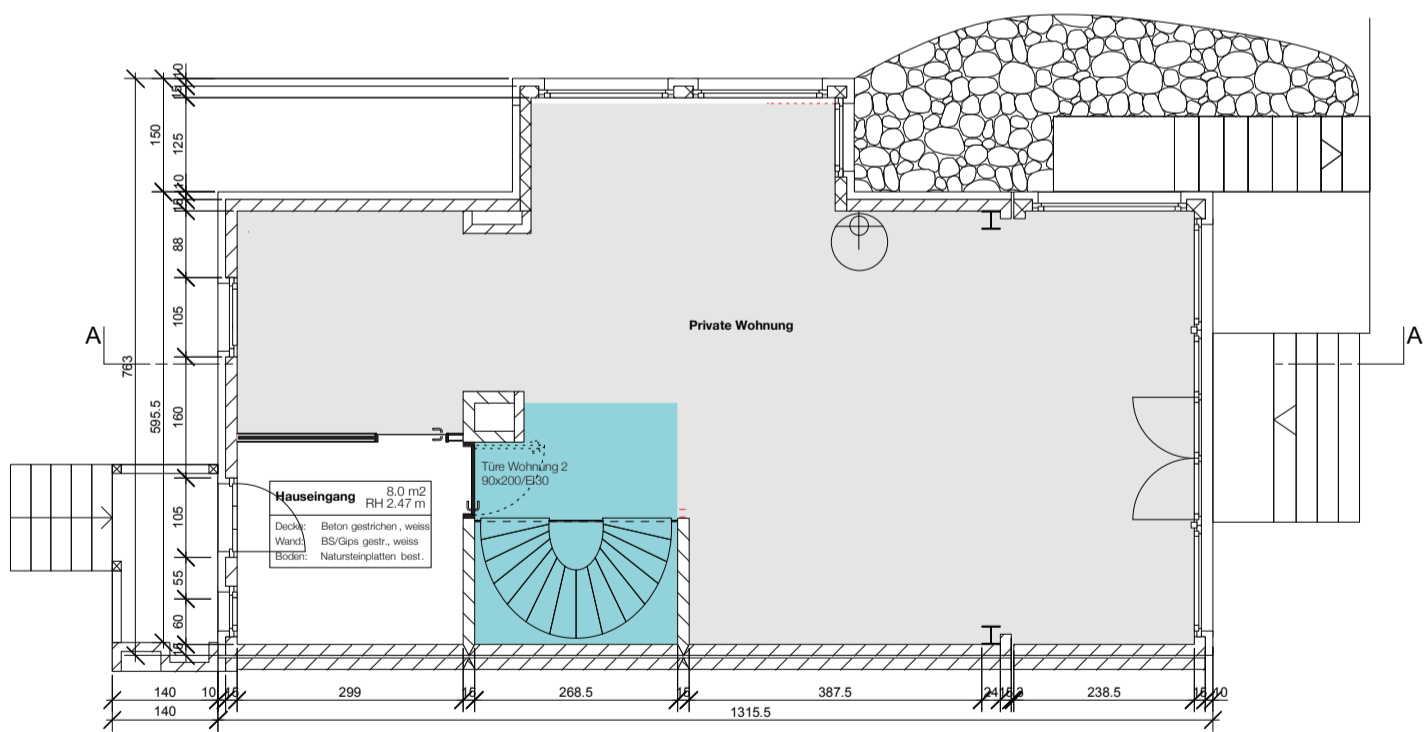
ERDGESCHOSS
