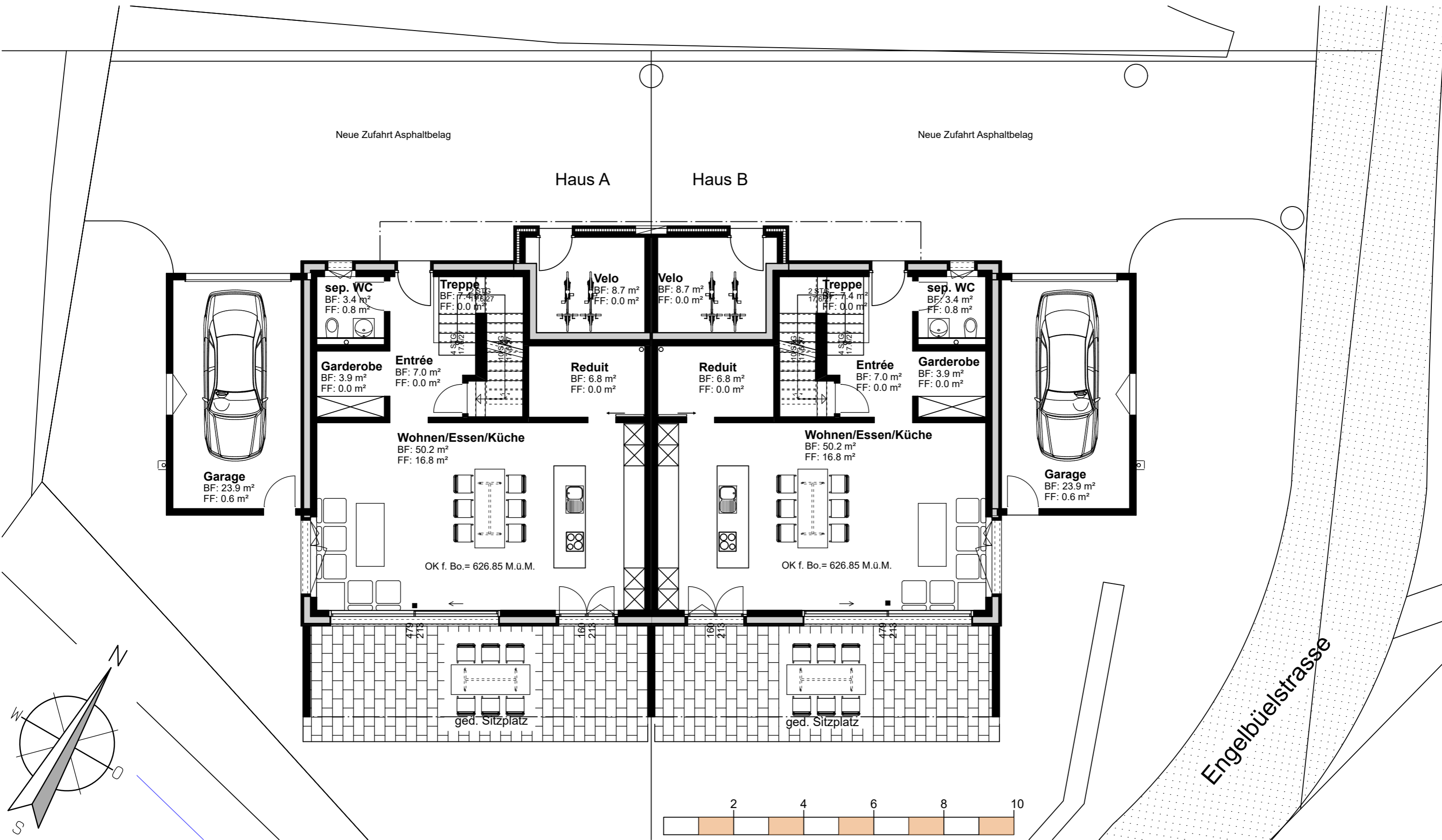
Grundriss Erdgeschoss
