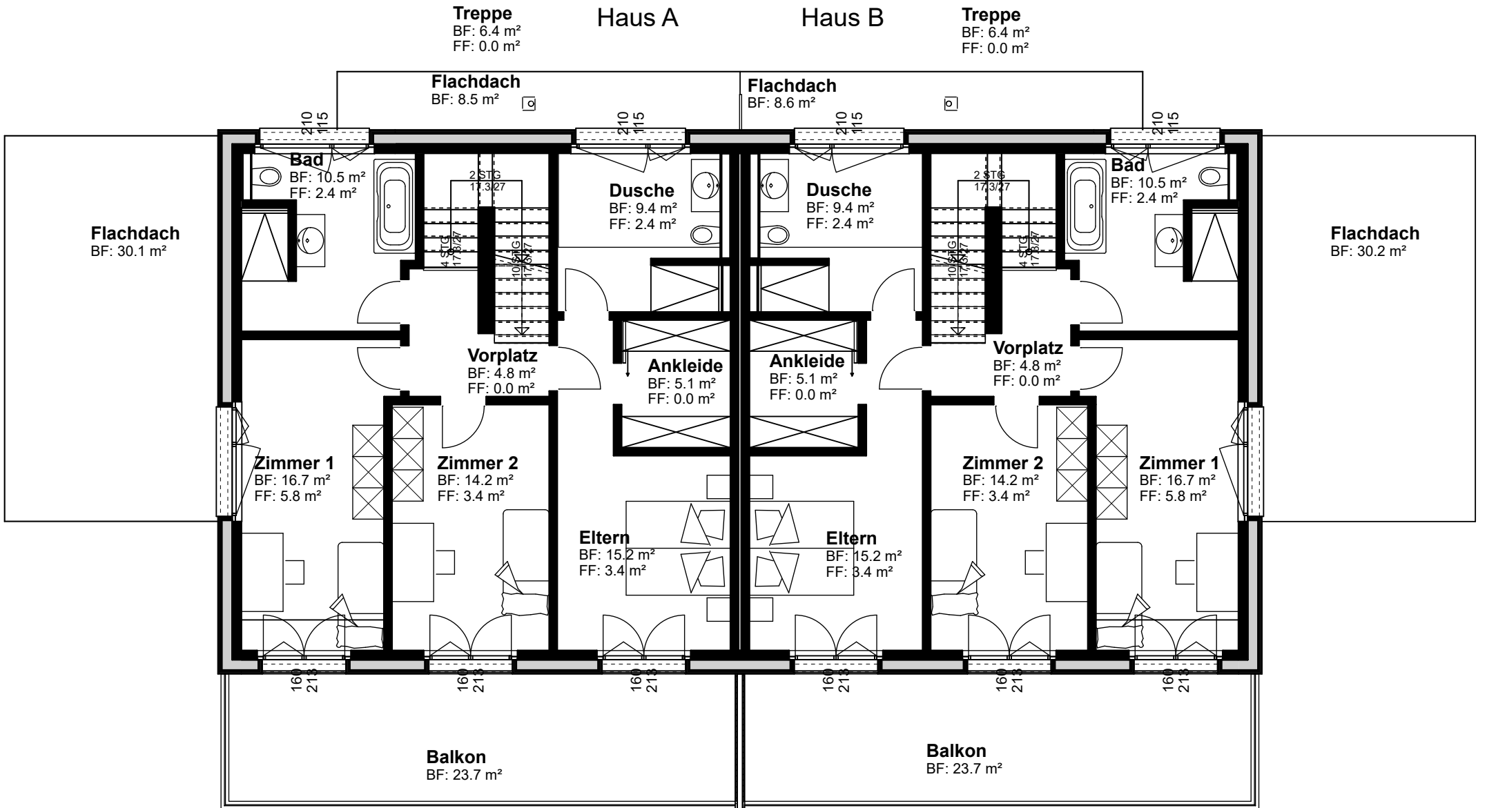
Grundriss Obergeschoss
