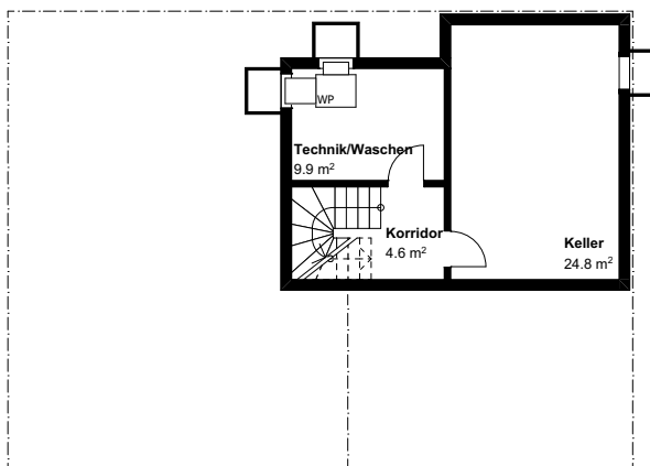
Untergeschoss
