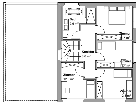
1. Obergeschoss
