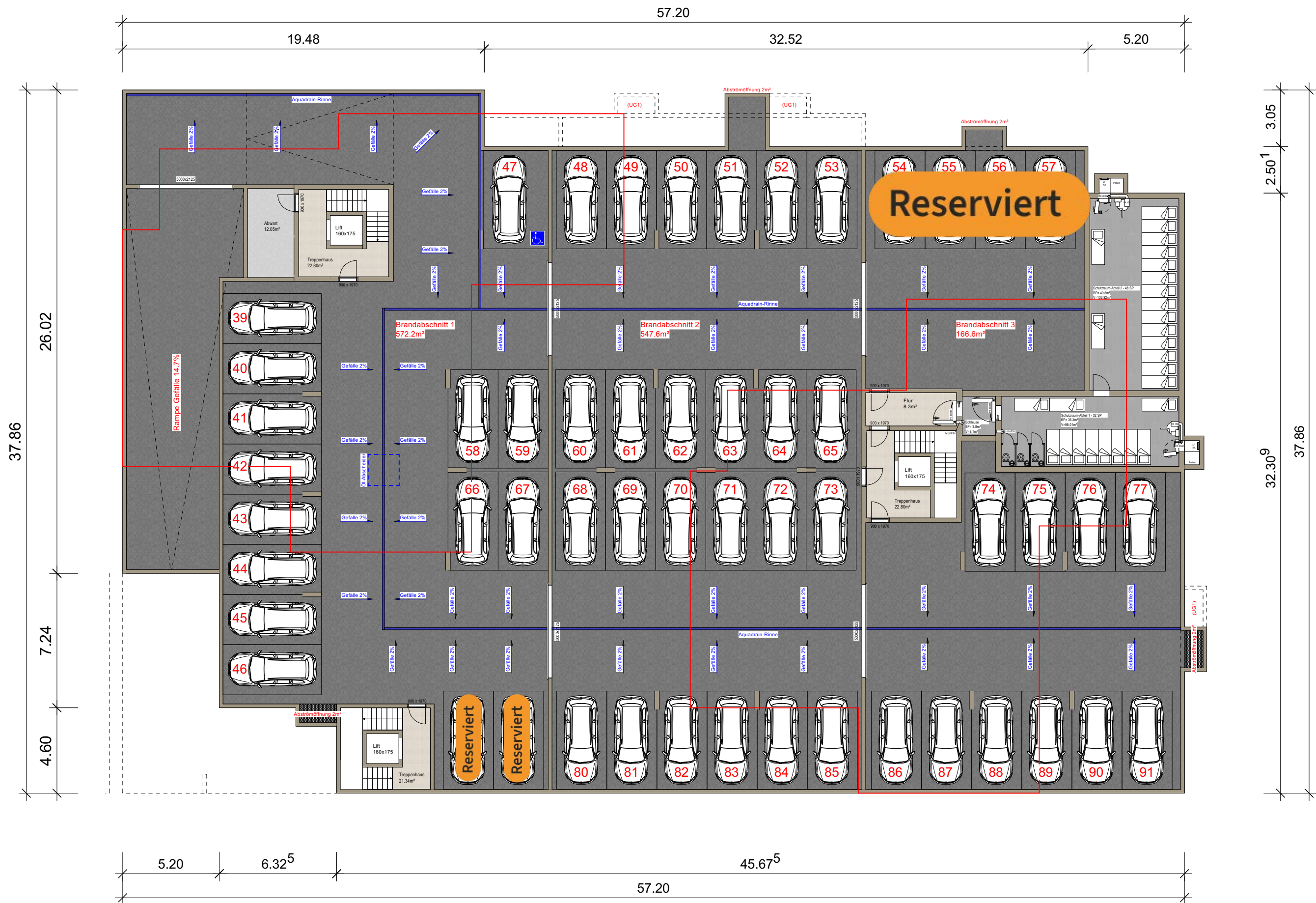
Grundriss 2.Untergeschoss MST:1:200
