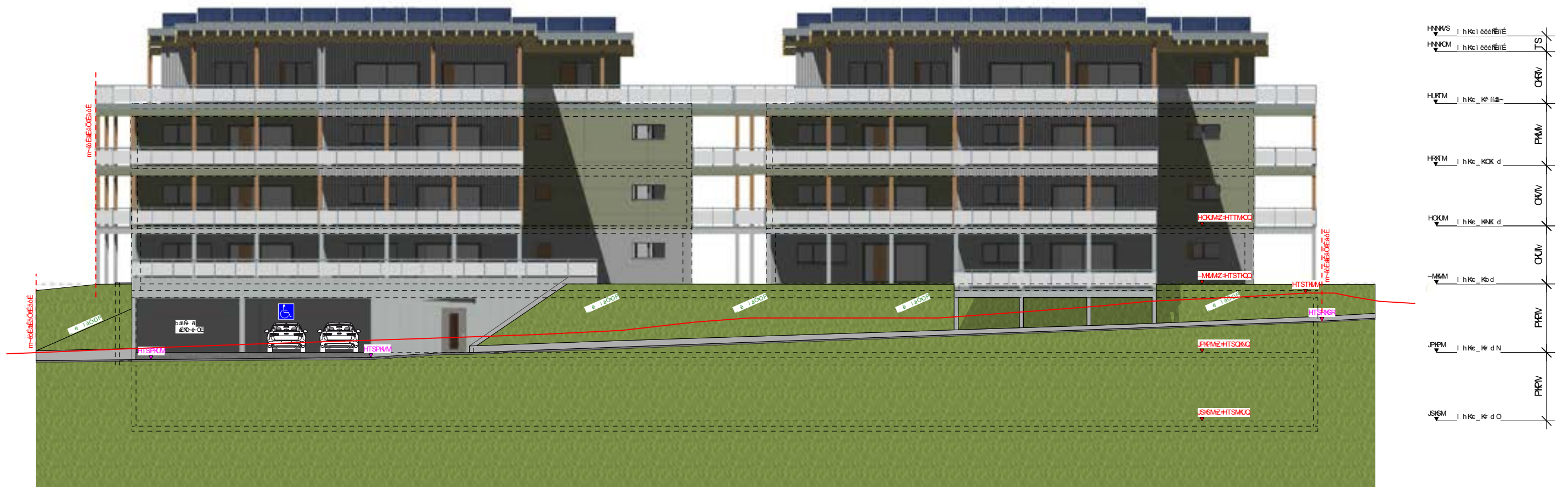
Fassade Süd-Ost MST:1:200
