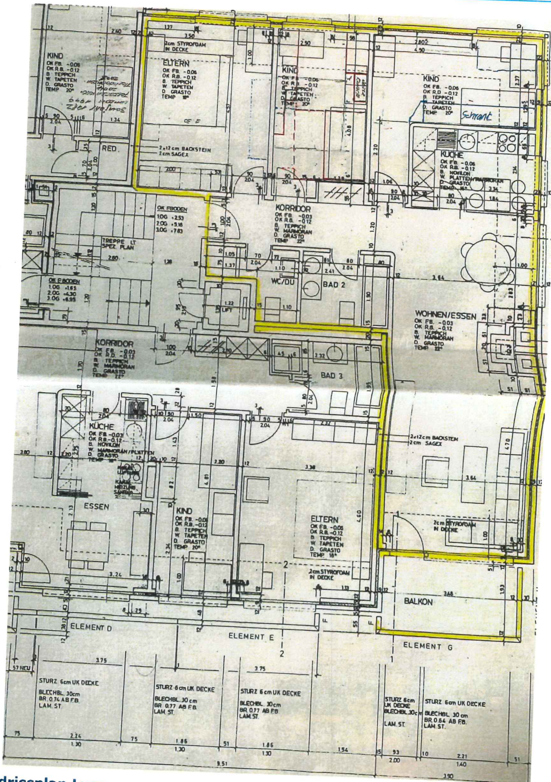
Grundrisplan Lyss
