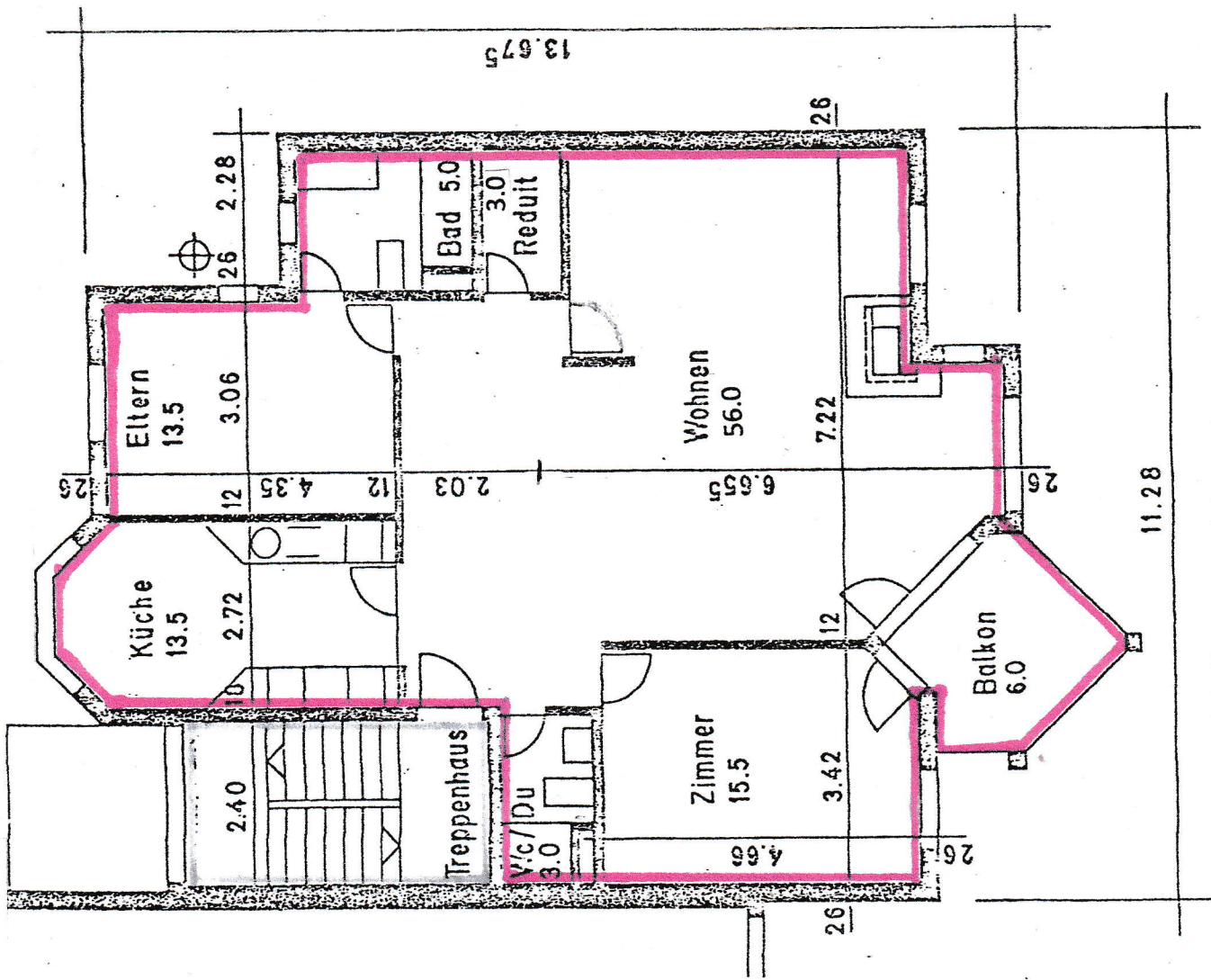
3,5 Zimmerwohnung 110 m2
