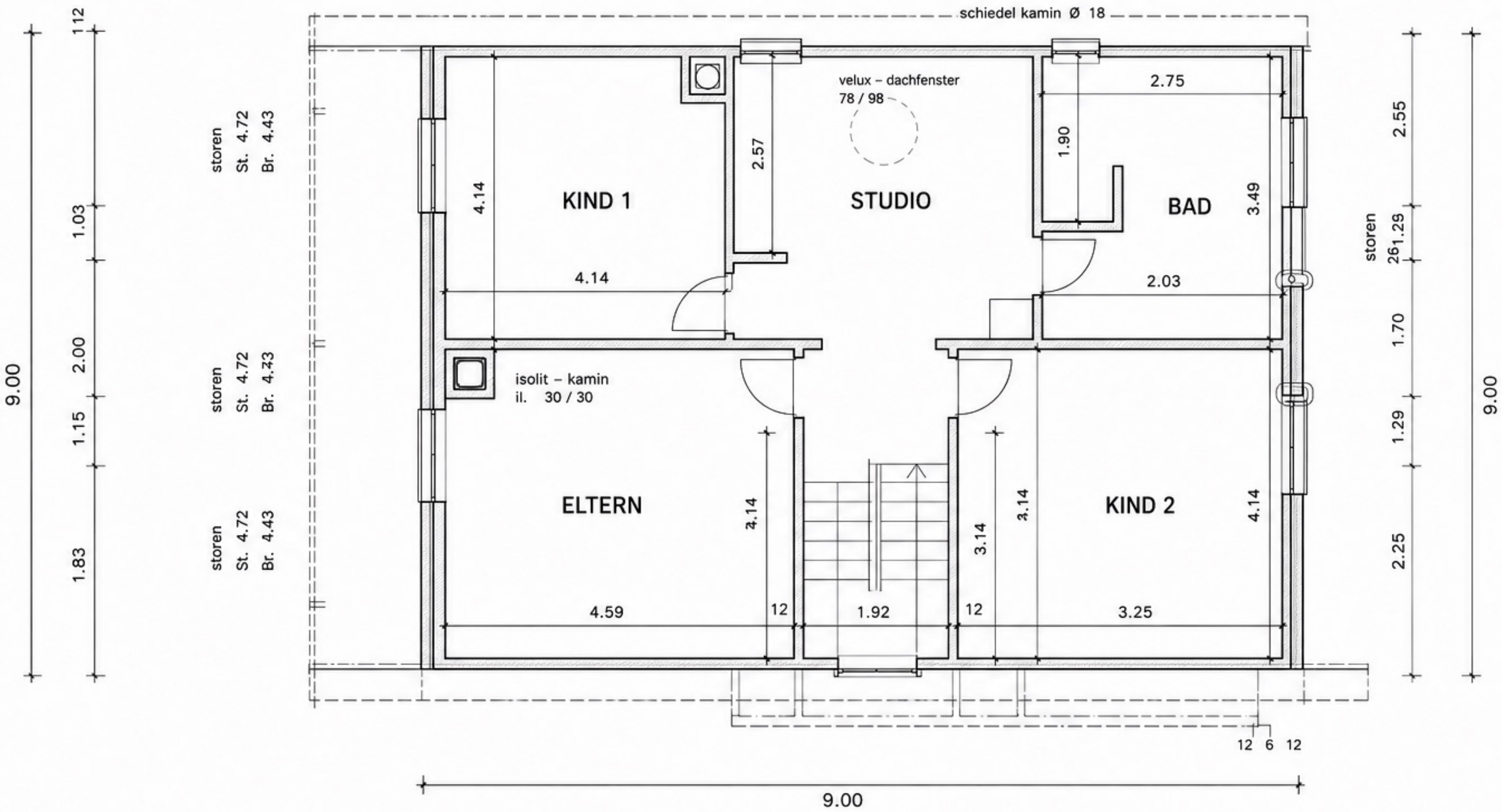
OBERGESCHOSS/DACHGESCHOSS MASSTAB 1:100
