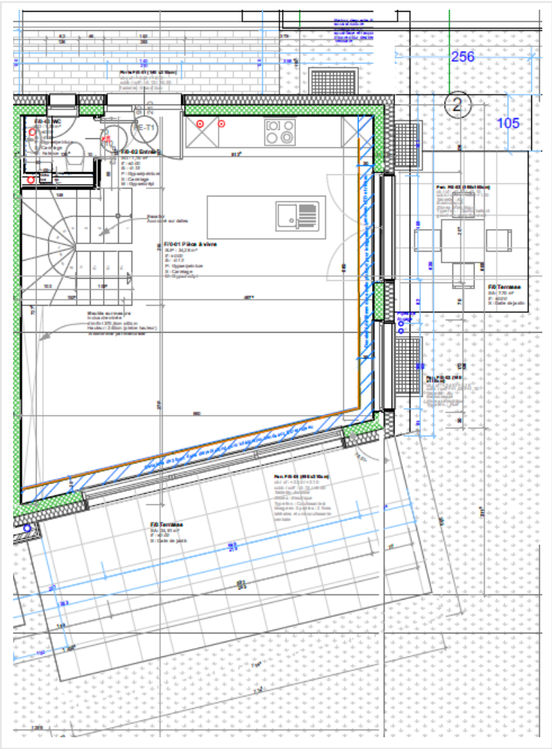
Rez-de-chaussée
