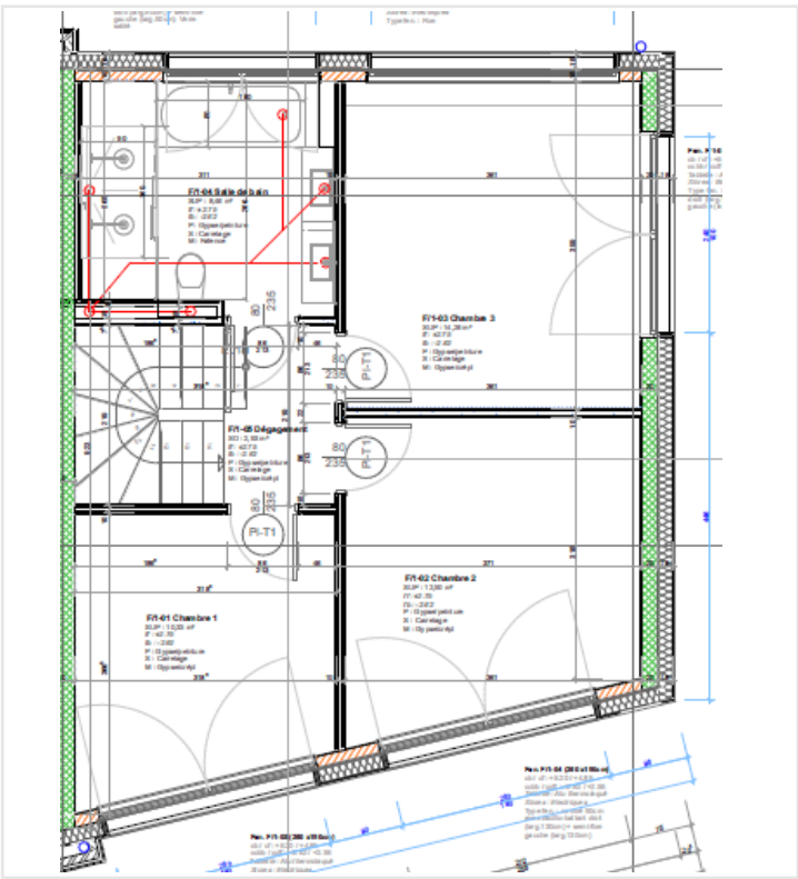
1 er étage
