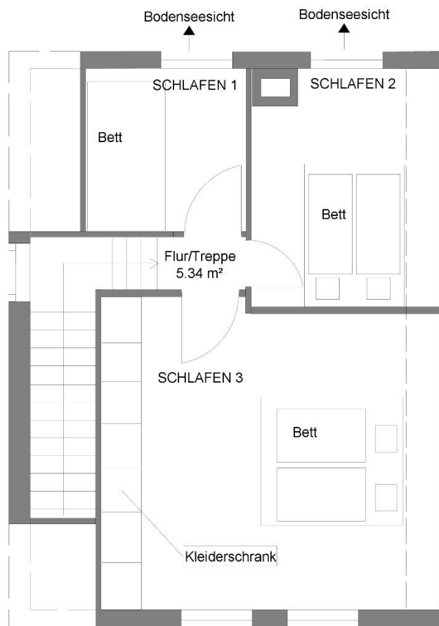
Dachgeschoss
