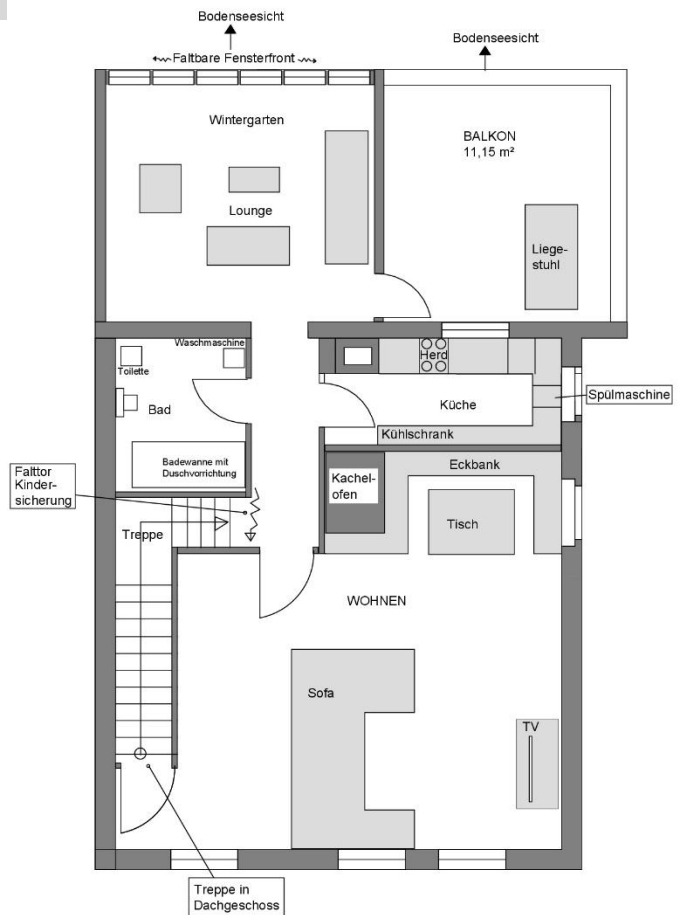
Erdgeschoss
