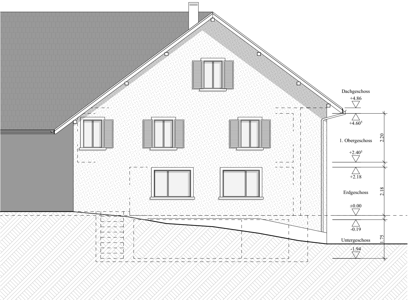
Nordfassade
