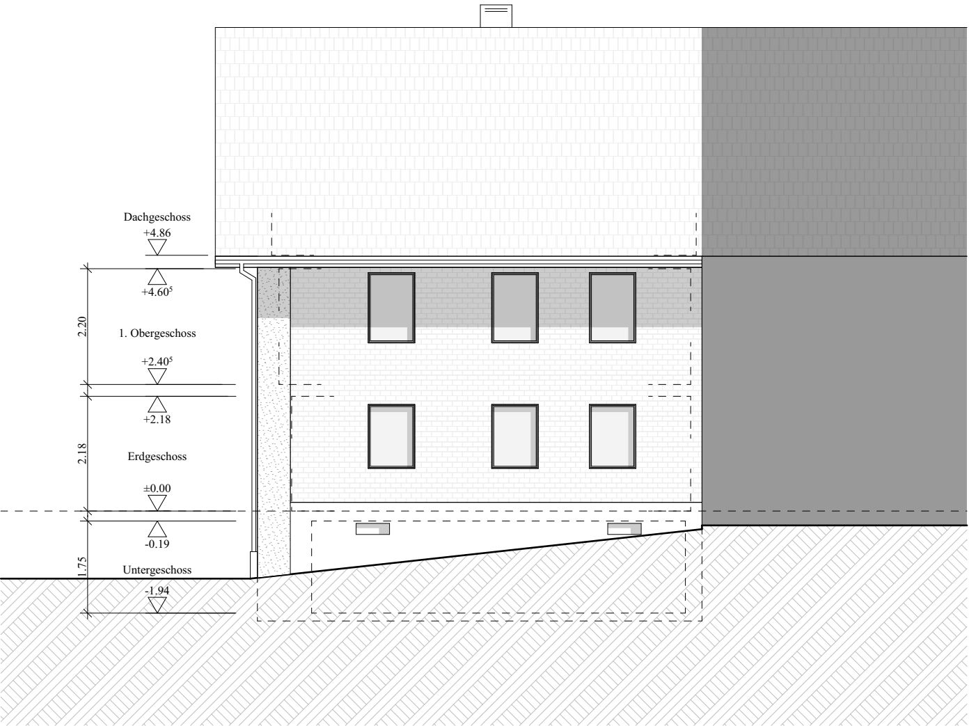
Südfassade
