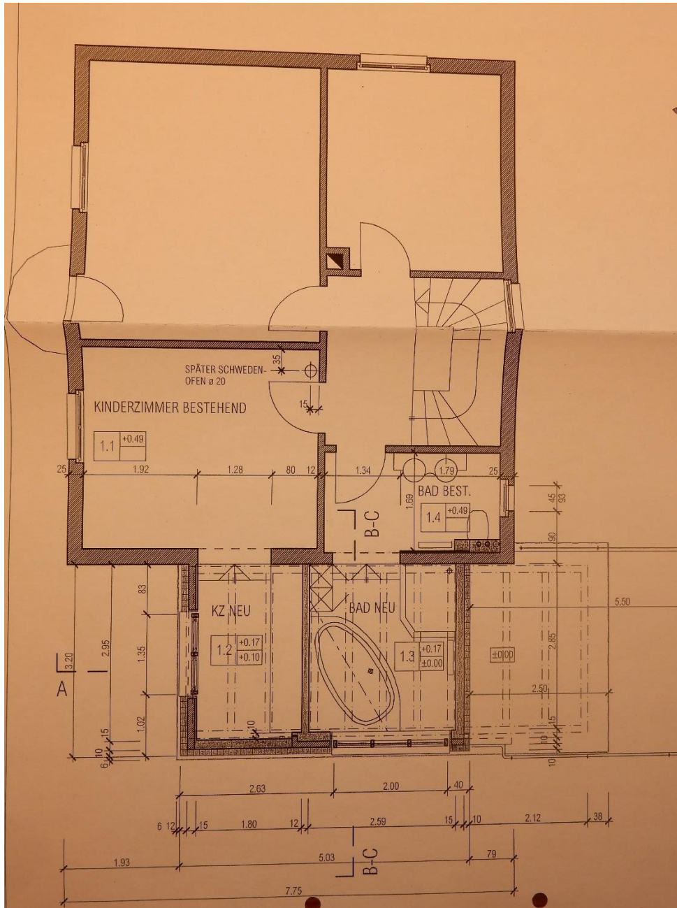
Grundriss erster Stock
