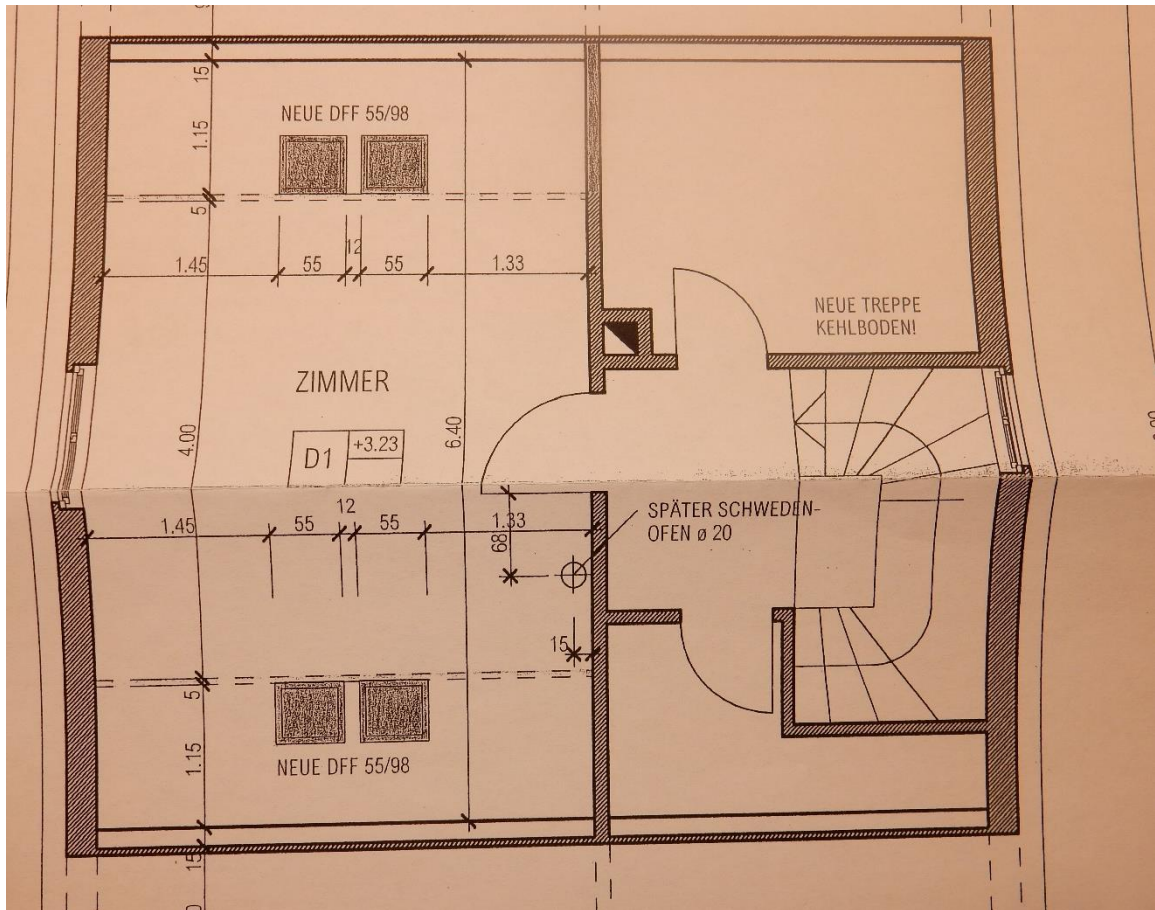
Grundriss Dachgeschoss
