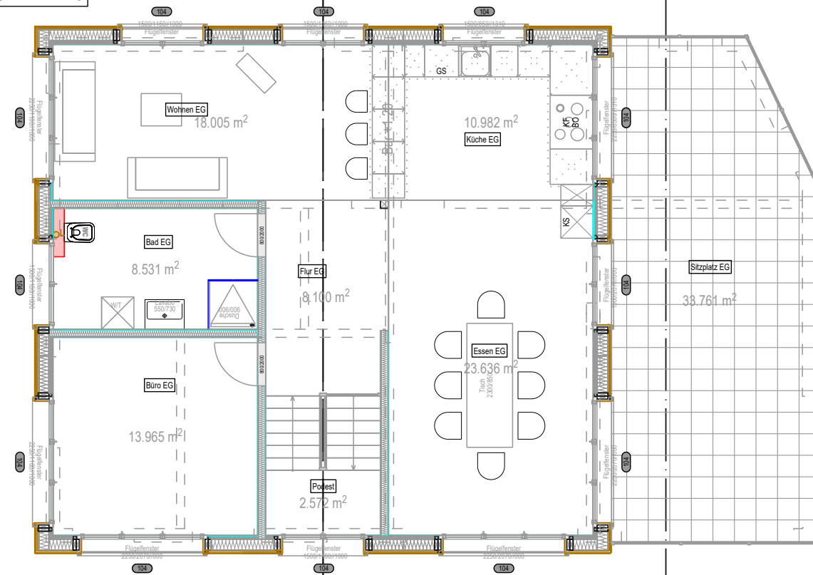
Grundriss EG
