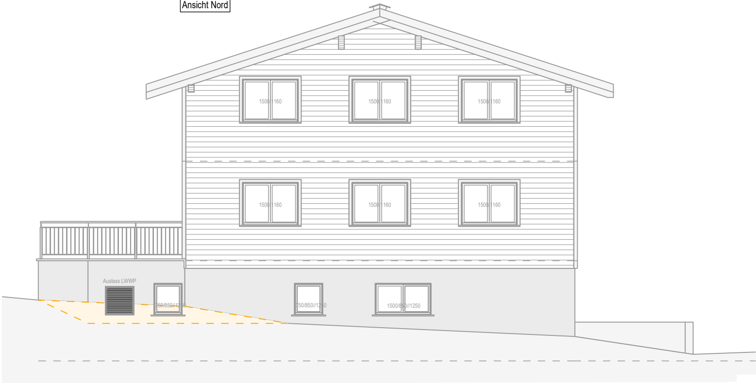
Ansicht Nord
