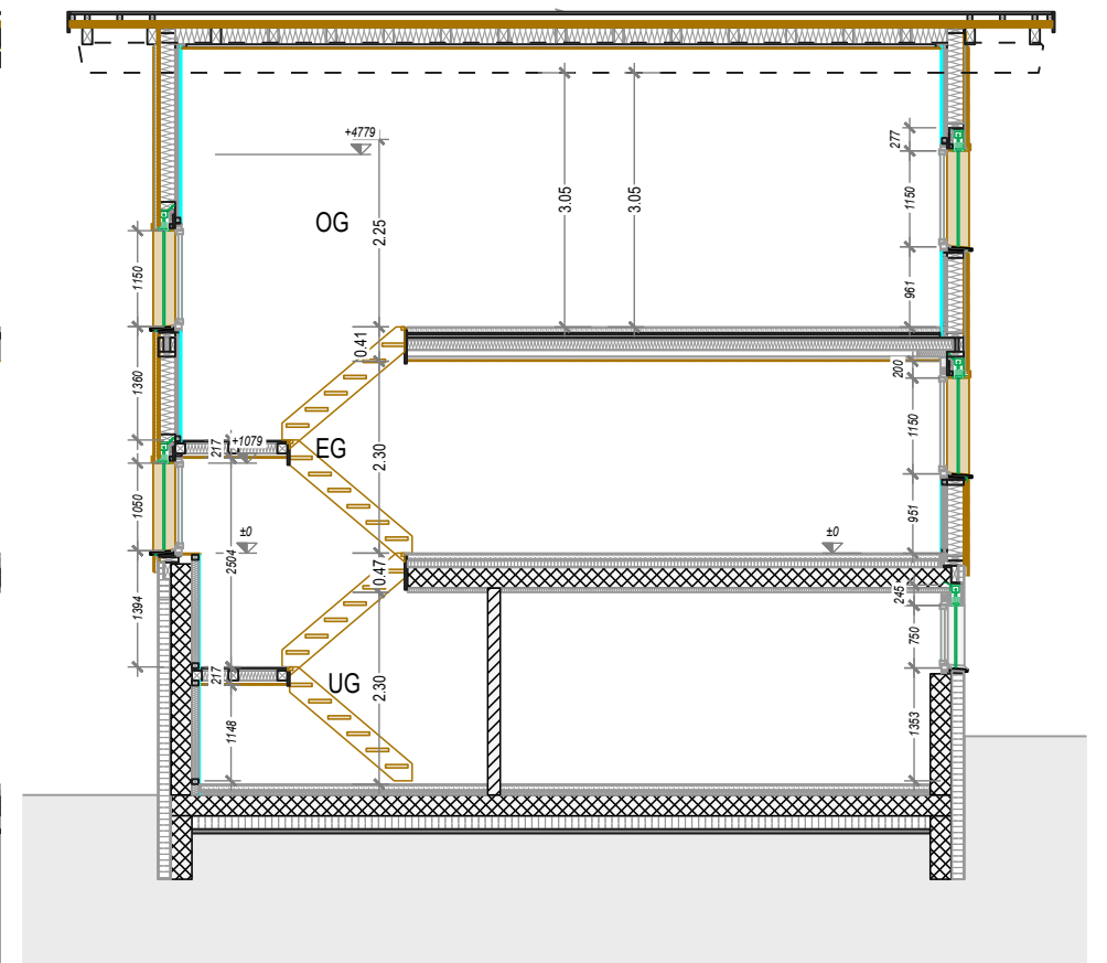
Schnitt 2-2
