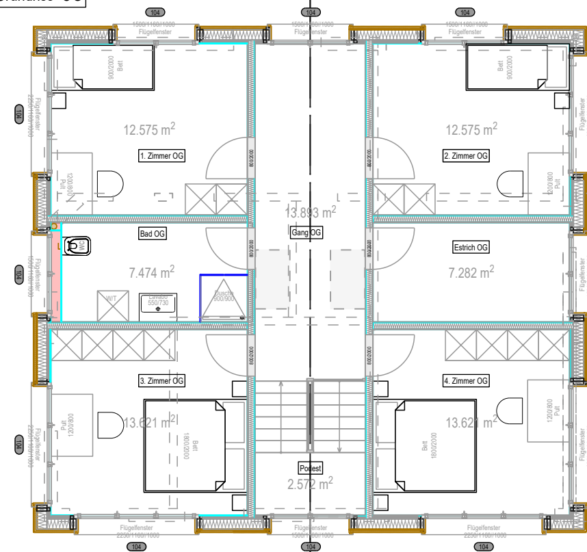
Grundriss OG
