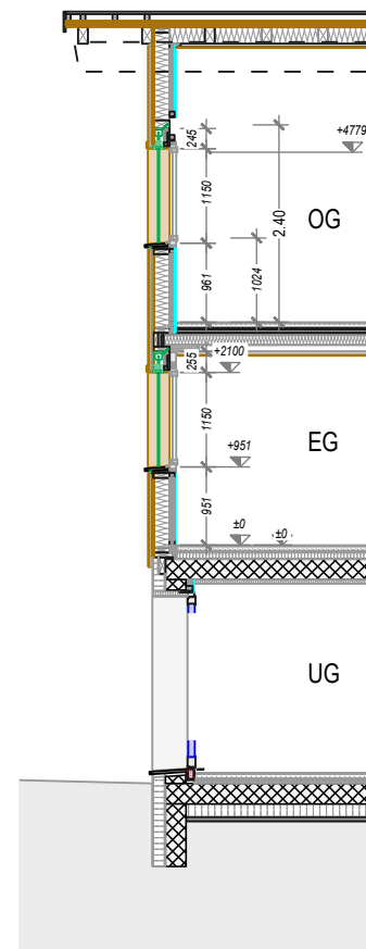
Schnitt 1-1
