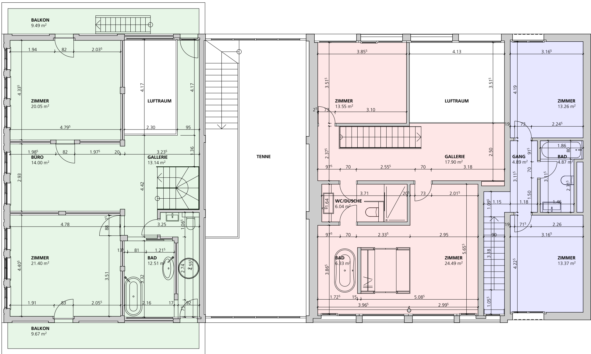
1. OBERGESCHOSS :
