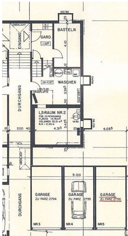
Kellergeschoss
