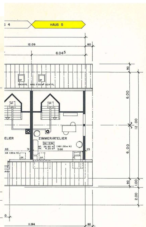
Galeriegeschoss
