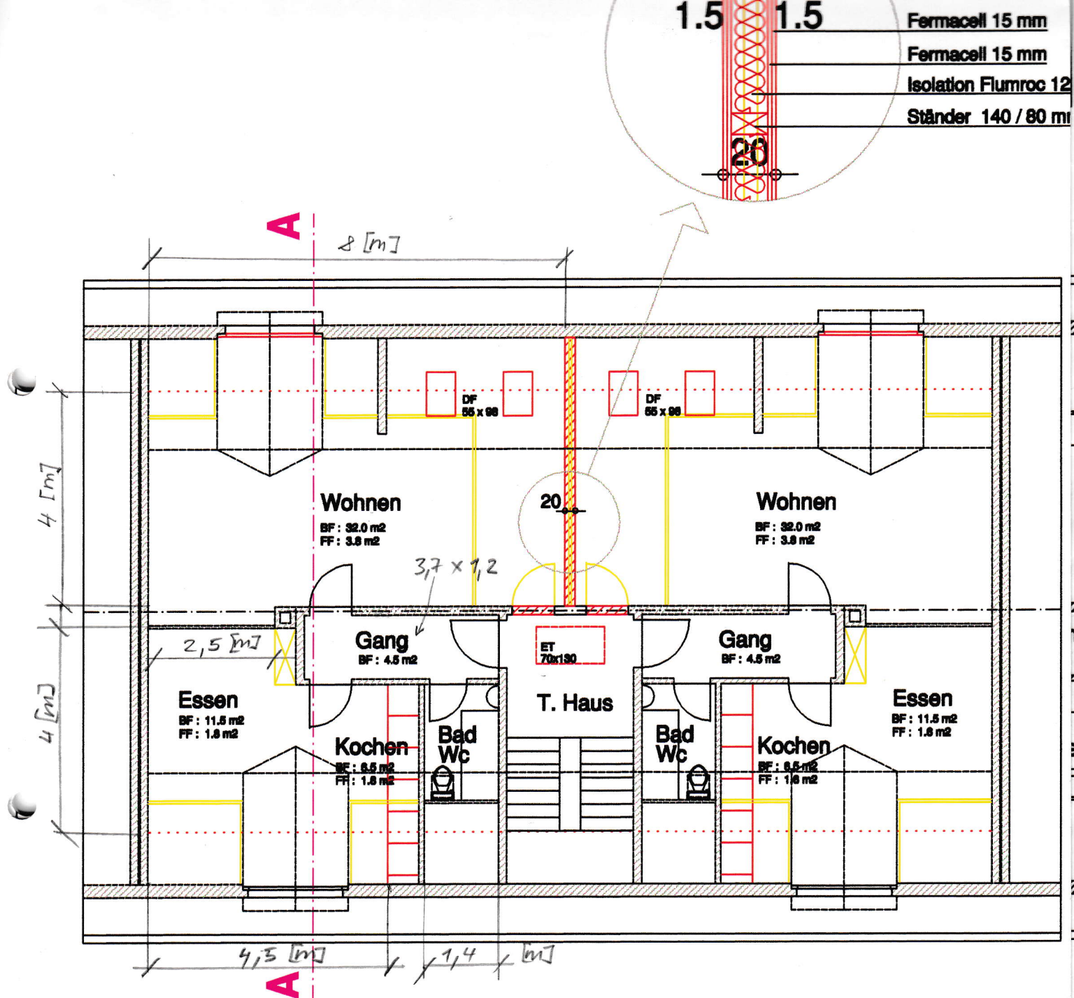
Grundriss Dachgeschoss
