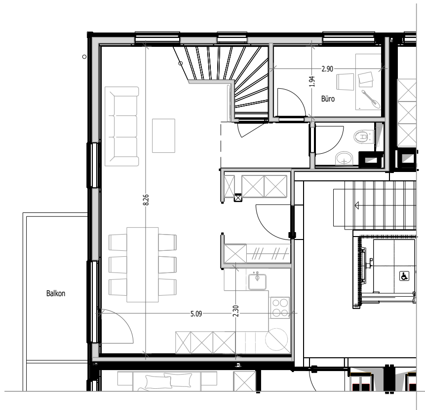
Dachgeschoss
