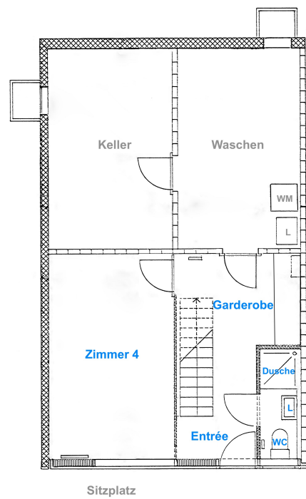
Grundriss Tiefparterre
