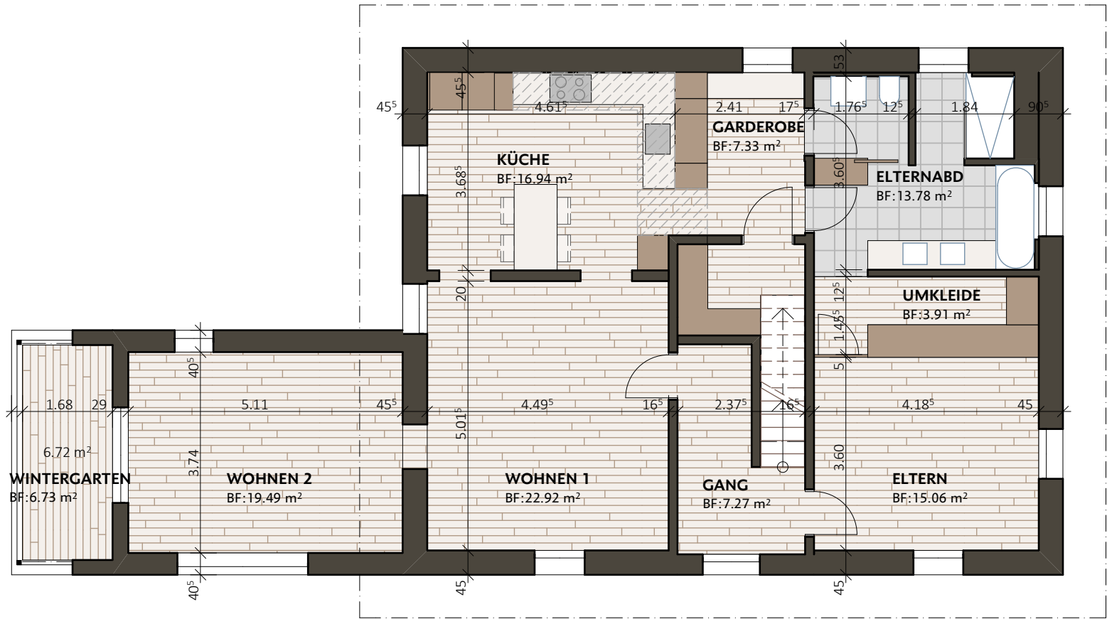
OBERGESCHOSS
