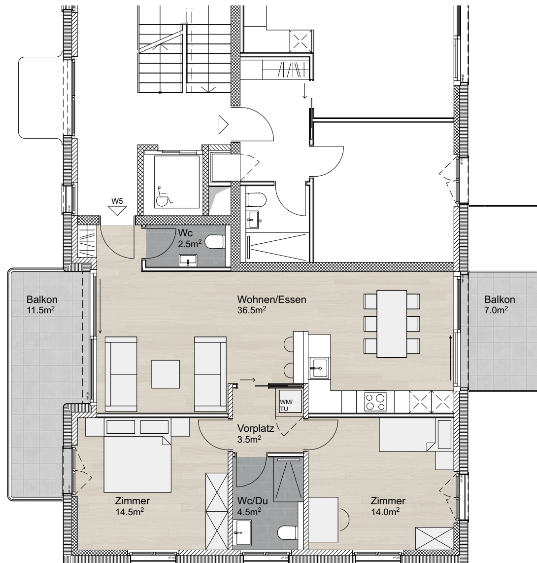
Grundriss Mst. 1:100
