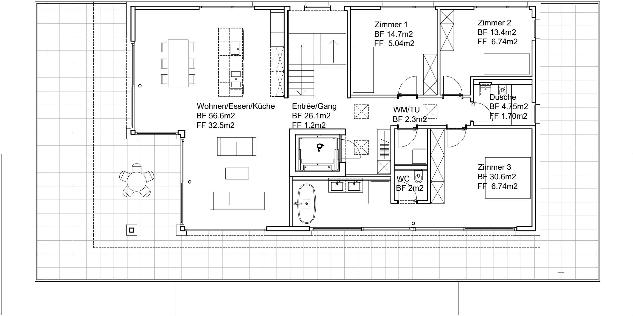
ATTIKA 4.5Zi-Wohnung NF 150.5m 2
