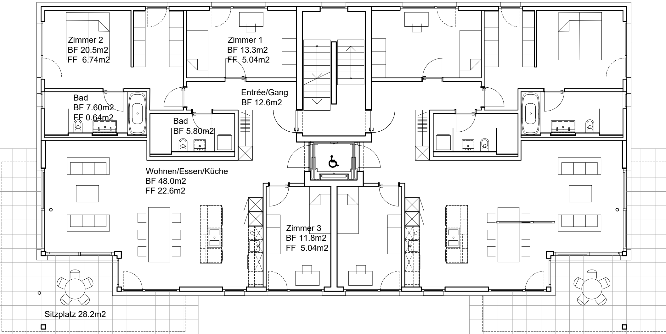
Erdgeschoss 4.5Zi-Wohnung NF 119.6m 2
