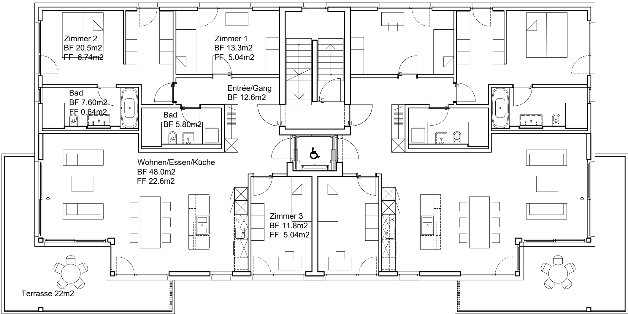
Obergeschoss 4.5Zi-Wohnung NF 119.6m 2
