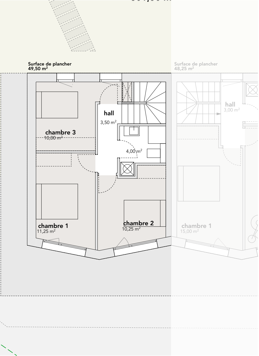
1er étage
