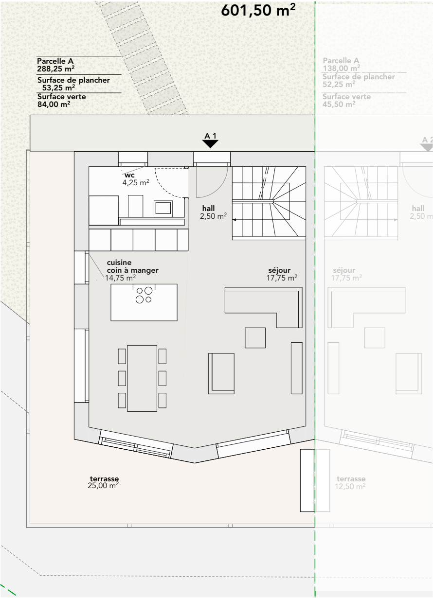
rez-de-chaussée
