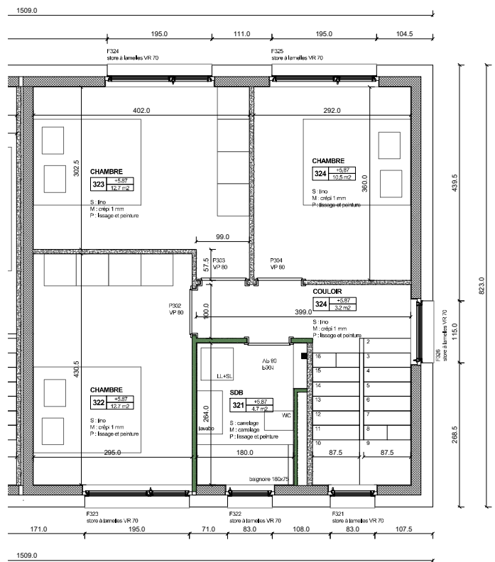
⌚ plan étage 2 _ 1:100
