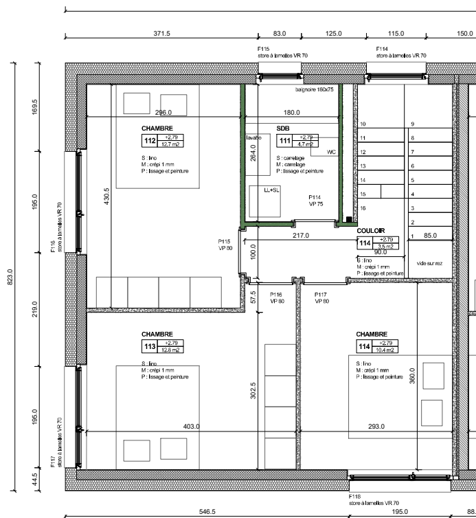
plan étage 1 _ 1:100
