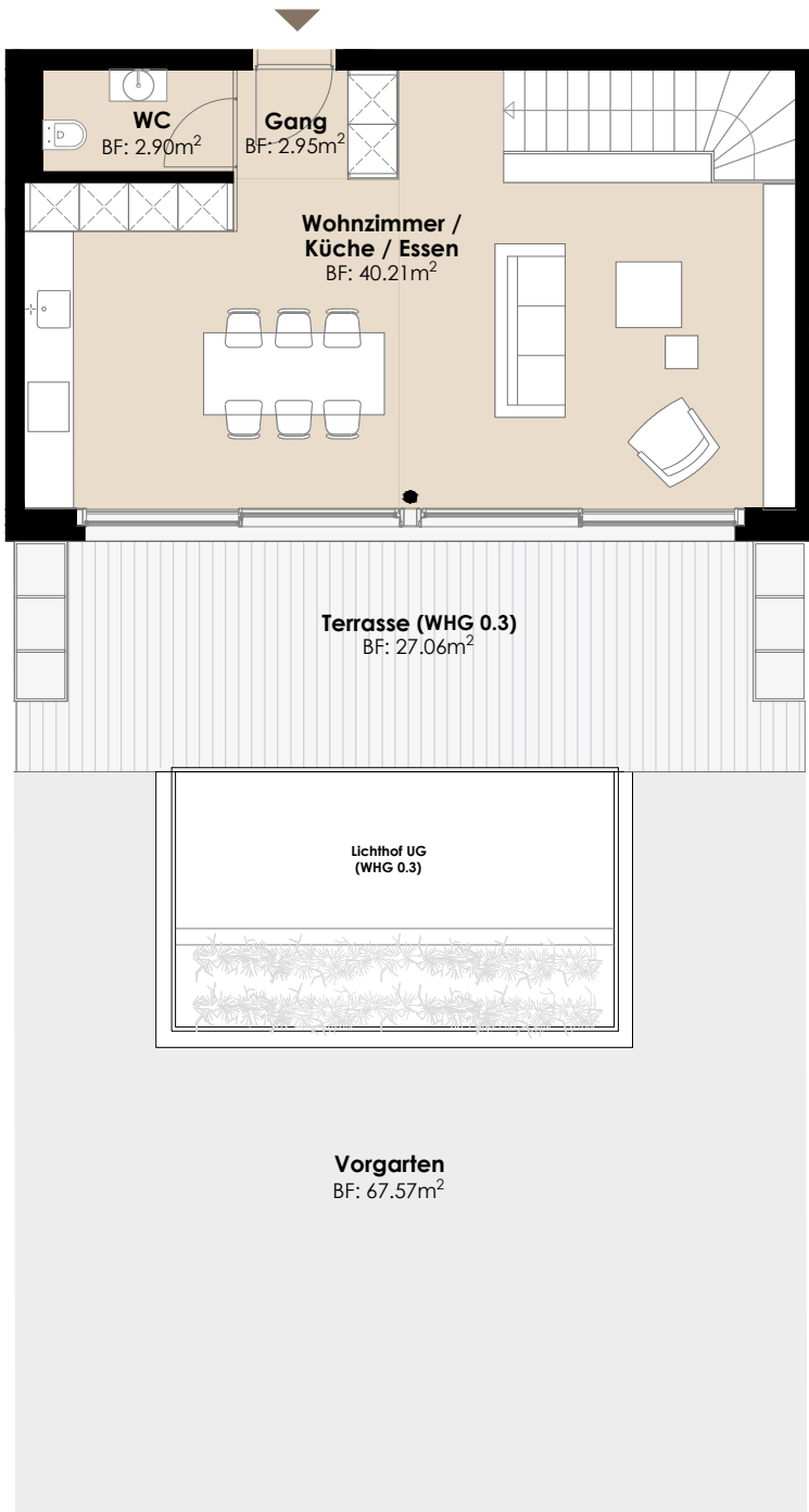
_Erdgeschoss
