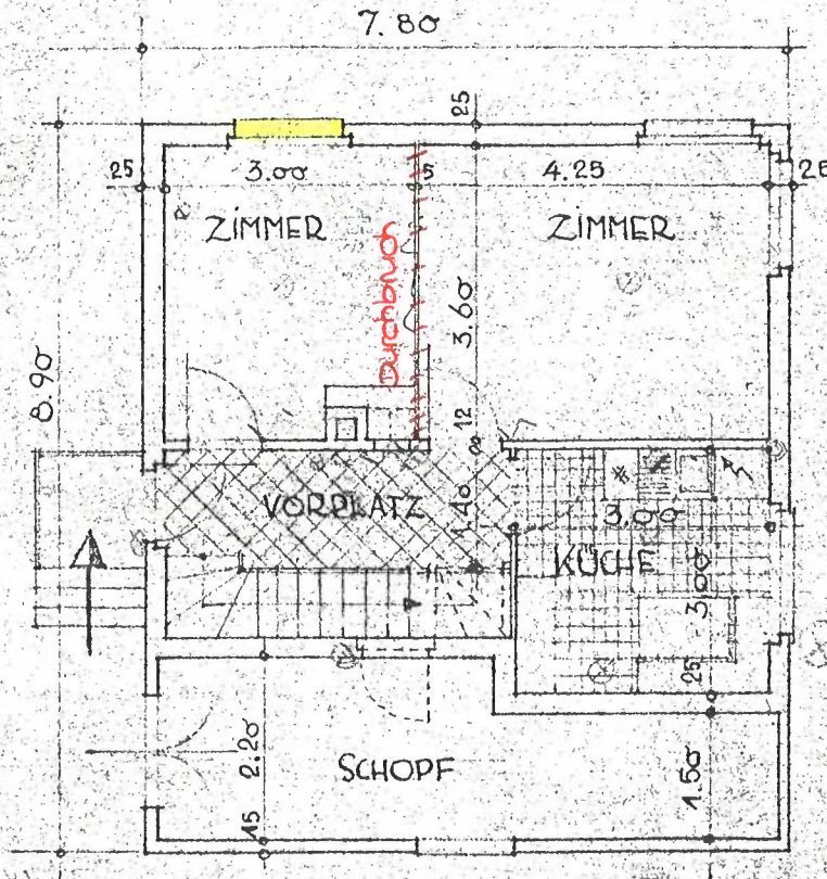
ERDGESCHOSS
