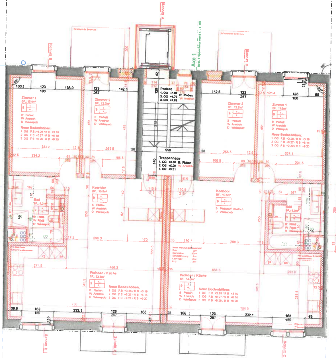
1.-3. Obergeschoss Werkplan
