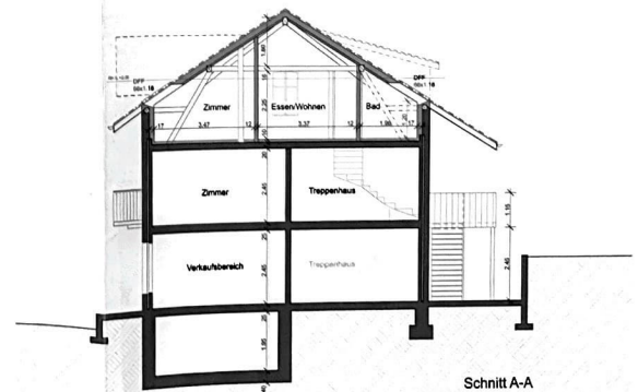
Schnitt A-A
