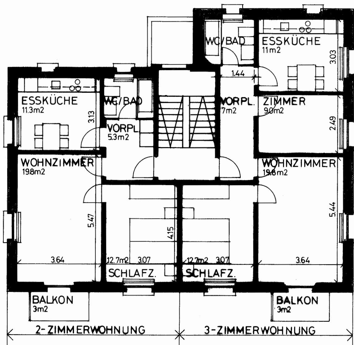
1. + 2. OBERGESCHOSS MST. 1:100
