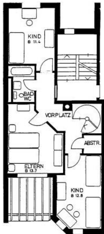
2. Obergeschoss
