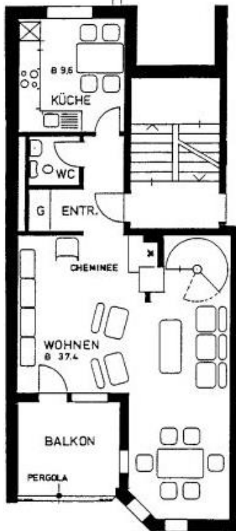
1. Obergeschoss
