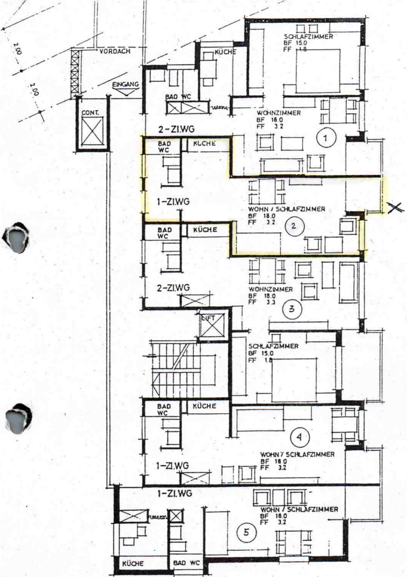
50 GESCHOSS E
