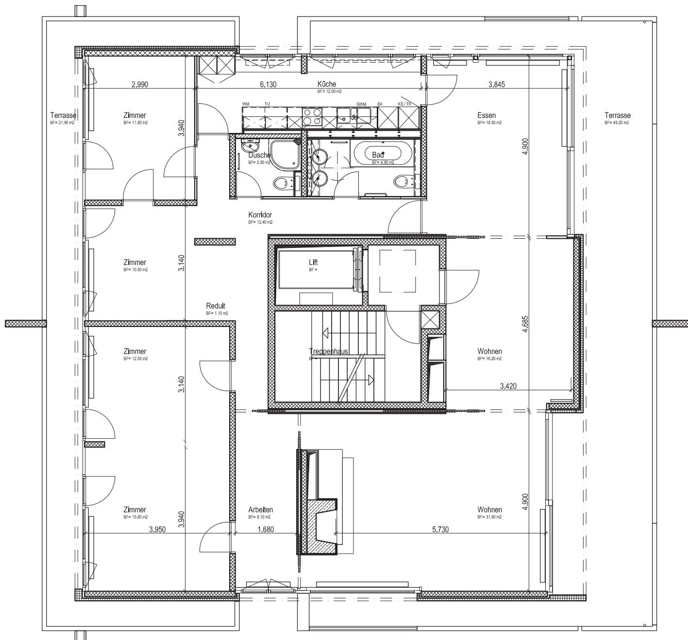
Grundriss 1:100
