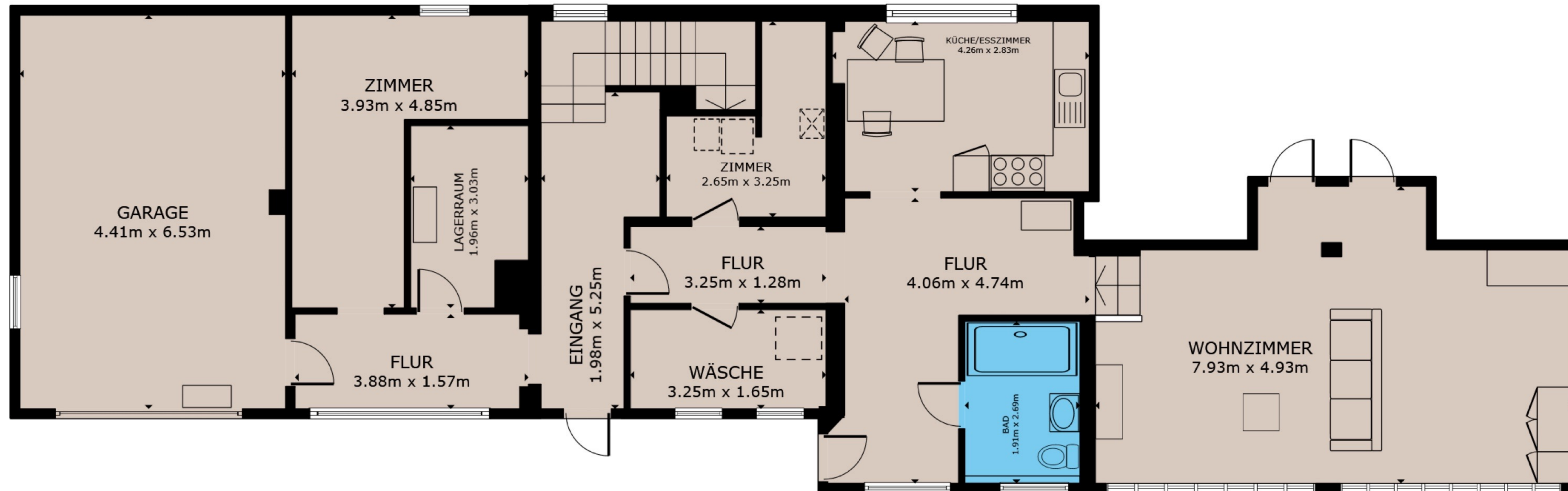
STOCKWERK 1
