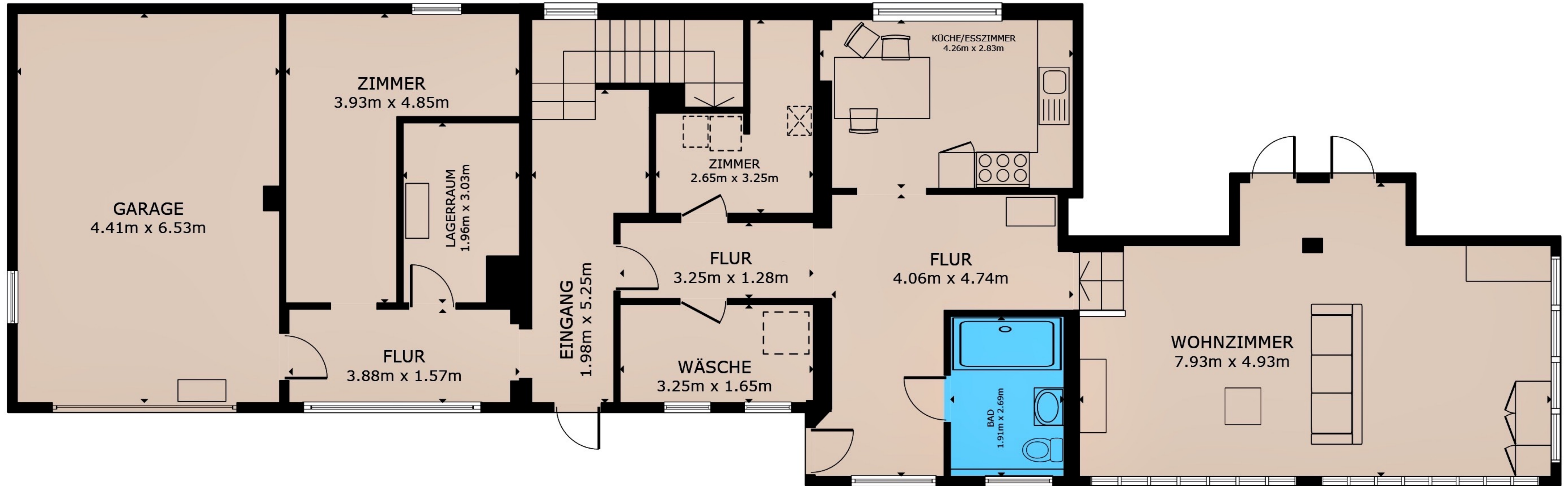
STOCKWERK 1
